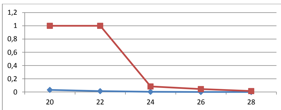
Фильтр Gaussian: M-fsk2 (красный) и 4 (синий)
