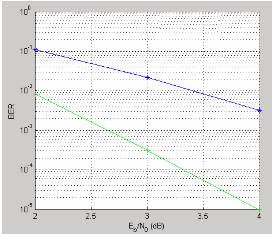
Рис. 3.97. График зависимости коэффициента битовых ошибок от отношения сигнала к шуму ( BER = f\left(\frac{E_s}{N_0}\right) ) для жесткого (синяя линия) и мягкого (зеленая линия) принятий решений сверточного декодирования последовательного метода Витерби.
