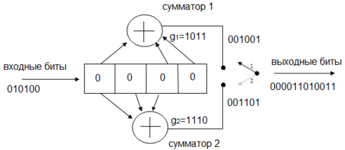
Рис. 3.85. Свёрточный кодер
