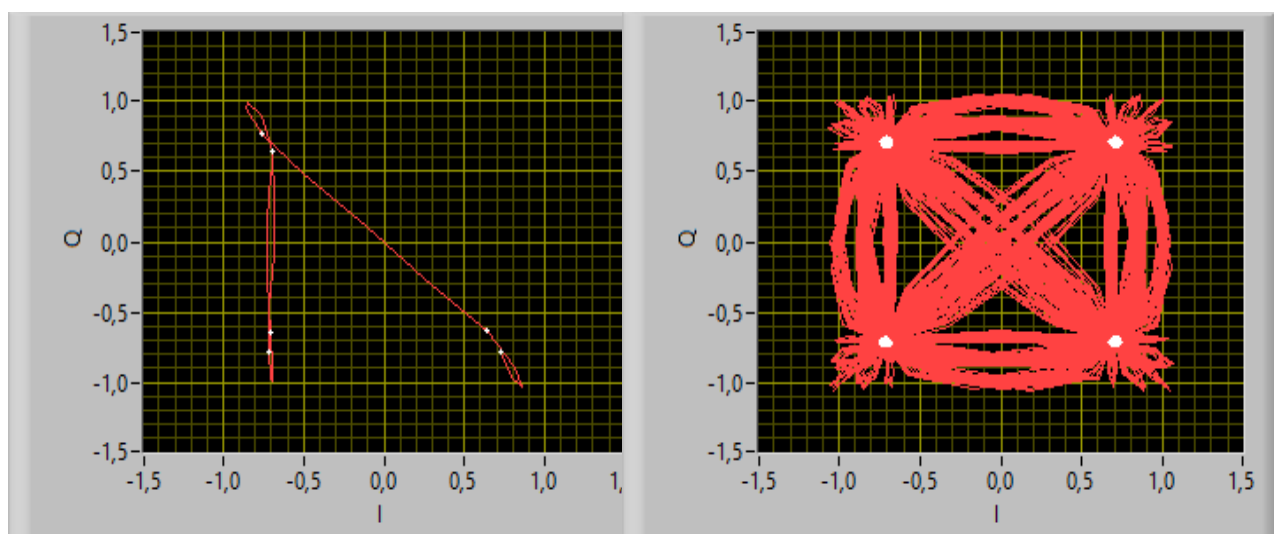
Рис. 1.65. Диаграмма QPSK. 10 символов в сообщении (слева), 1000 символов в сообщении (справа).
