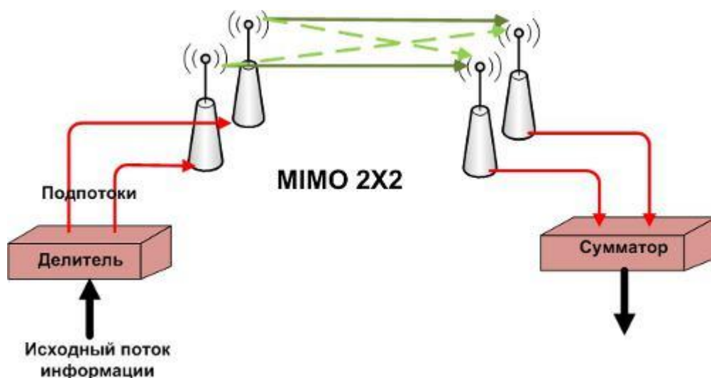
Рис. 4.28. Принцип организации технологии MIMO
