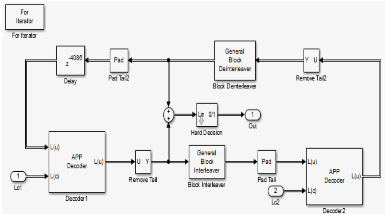
Рисунок 3.154. Схема турбо-декодера
