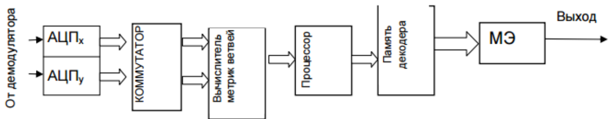
Рис. 5.20. Структурная схема декодера сверточного кода.
