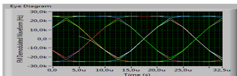
Рис. 1.28. Глазковая диаграмма
