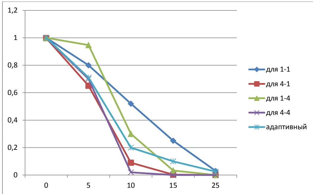
Рис. 4.34. Зависимость вероятности ошибок от отношения сигнал/шум
