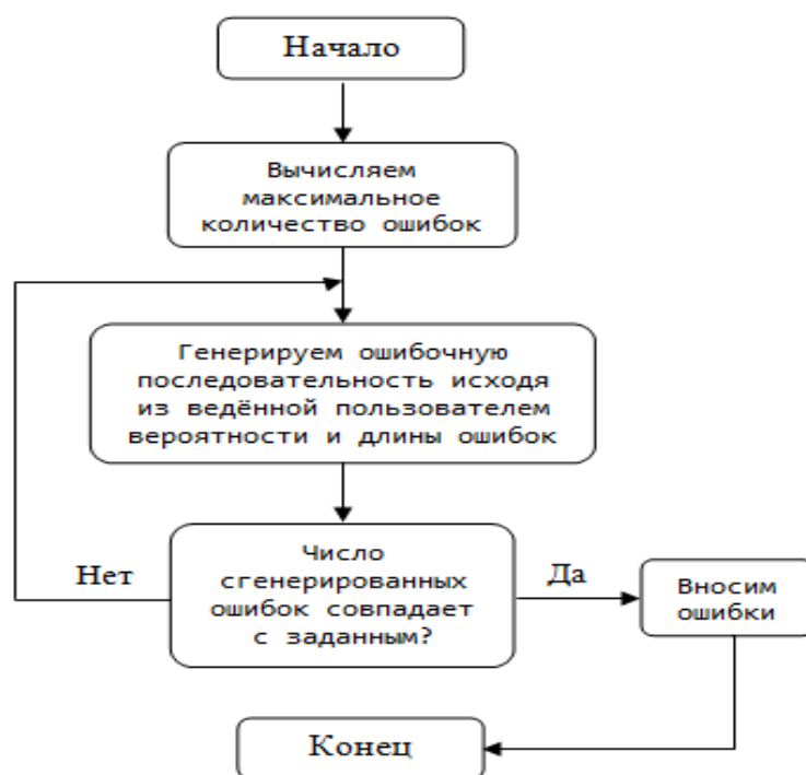
Рис. 3.77. Блок-схема для алгоритма имитации канала связи
