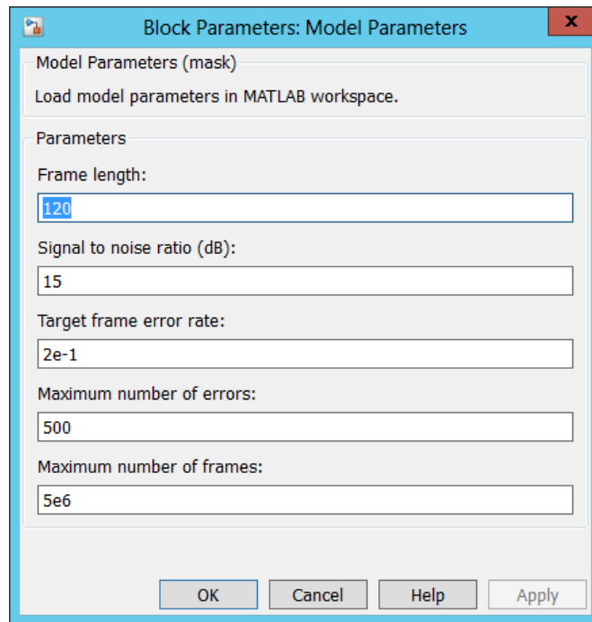
Рис. 4.30. Настройка блока канала
