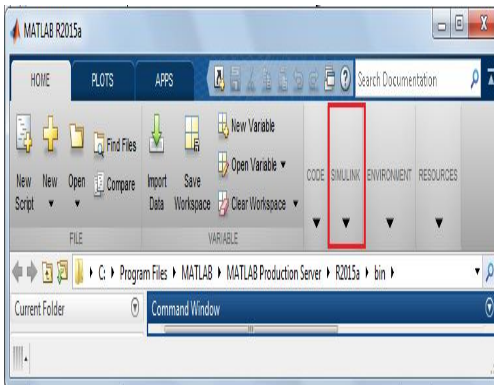
Рис. 4.10. Панель MATLAB
