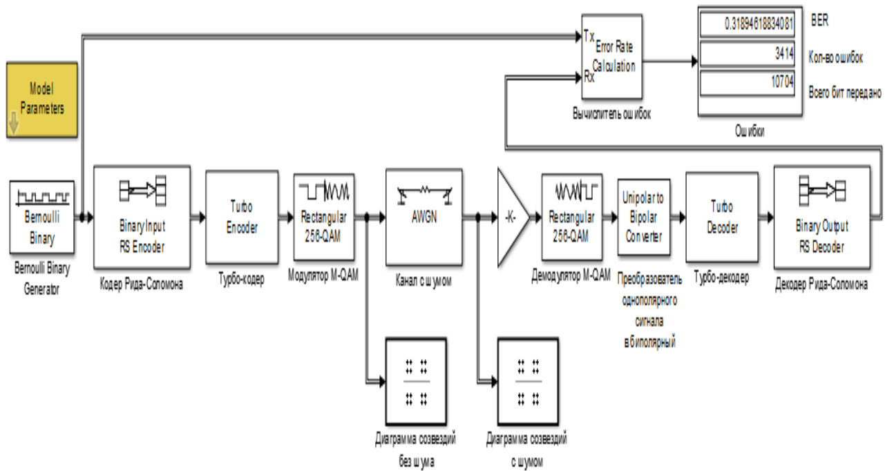
Рис. 3.143. Разработанная модель исследования каскадных кодов
