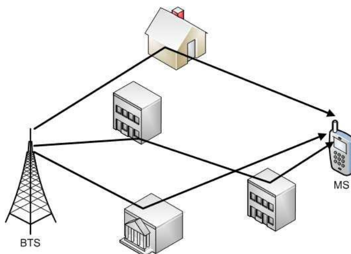
Рис. 4.26. Пример многолучевого распространения сигнала.
