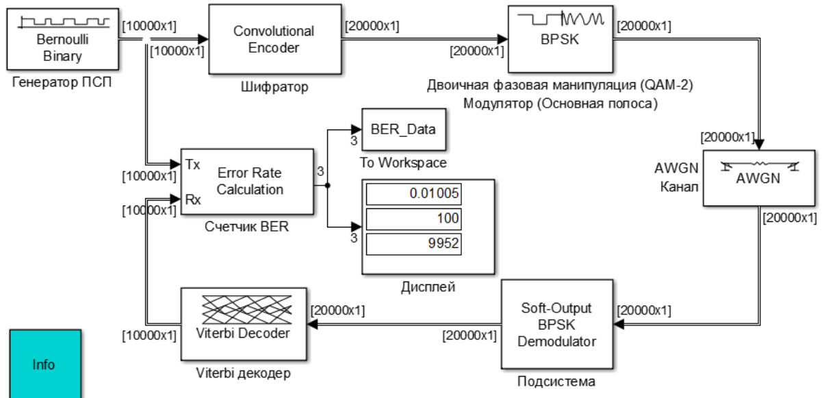
Рис. 3.95. Модель сверточного декодера Витерби при «Мягком решении»
