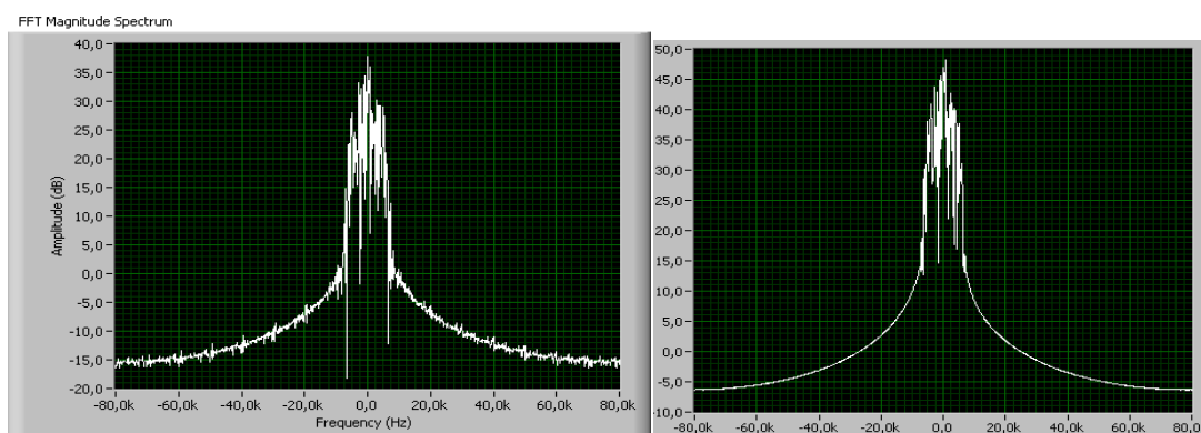
Рис. 1.83. Спектрограммы на входе и на выходе канала
