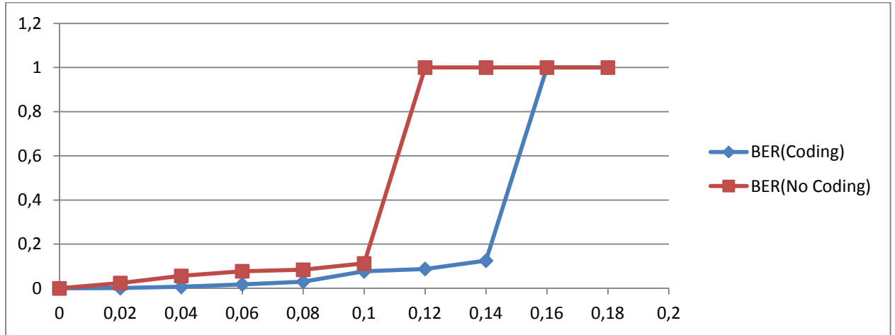
Рис. 3.122. График зависимости BER от Noise
