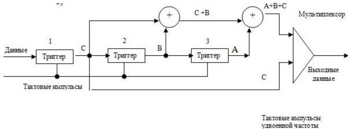
Рис. 5.14. Структурная схема кодера
