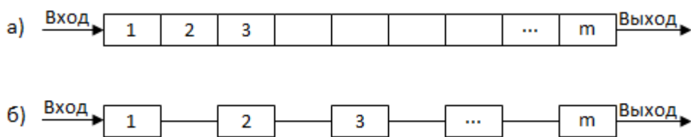
Рис. 3.64. Регистр сдвига
