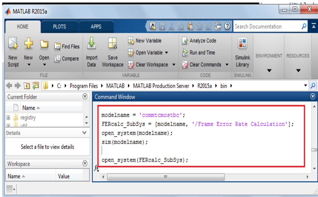
Рис. 4.6. Панель MATLAB 2015
