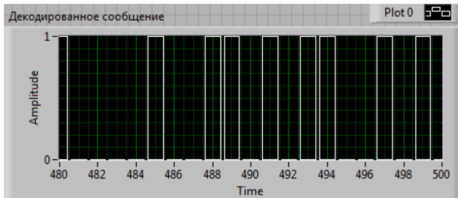
Рис. 3.126. Декодированное сообщение
