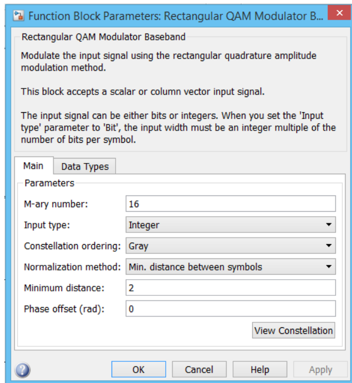
Рис. 4.43. Настройки QAM – модулятора
