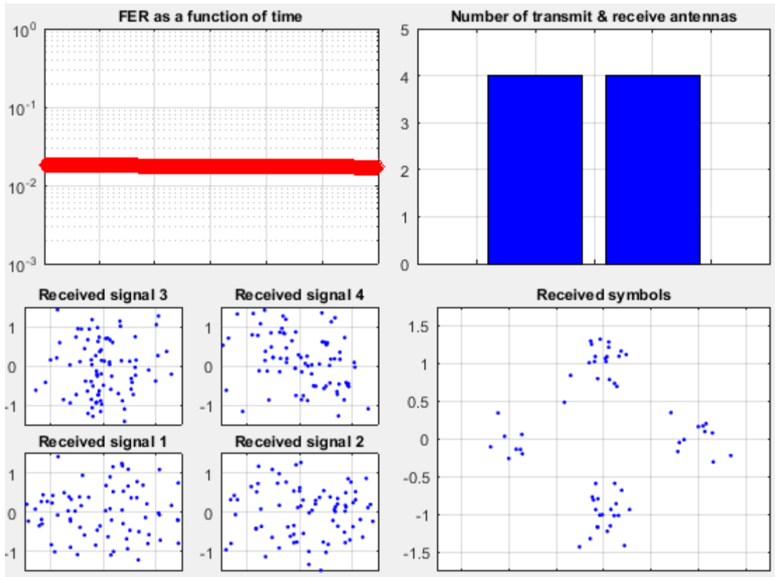
Рис. 4.60. Работа блока Signal Visualization (MIMO: 4 передатчика -4 приёмник)
