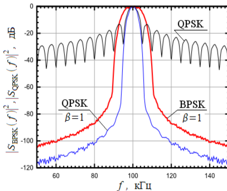
Рис. 1. 59. Спектр QPSK сигнала с формирующим фильтром Найквиста
