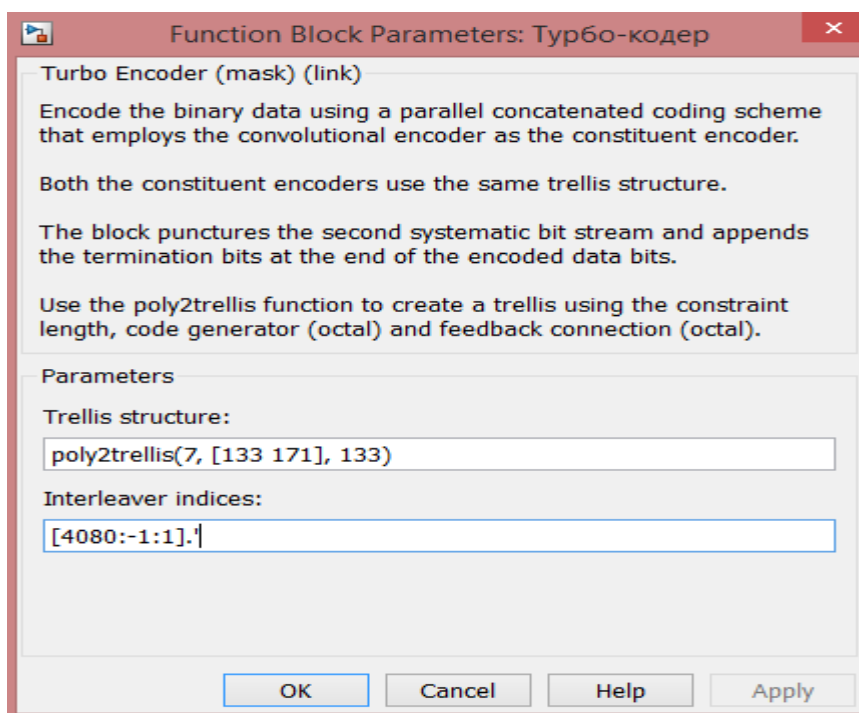
Рис. 3.147. Параметры блока «Turbo Encoder»
