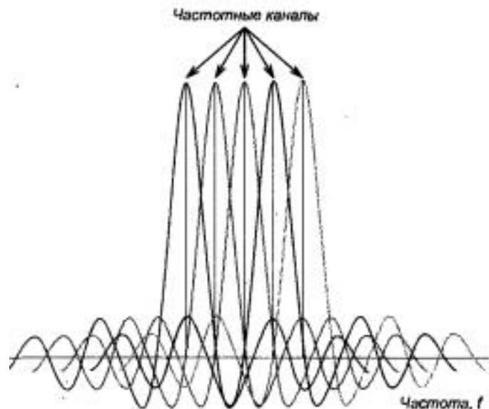
Рис. 4.26. Частотное разделение каналов с ортогональными несущими сигналами.
