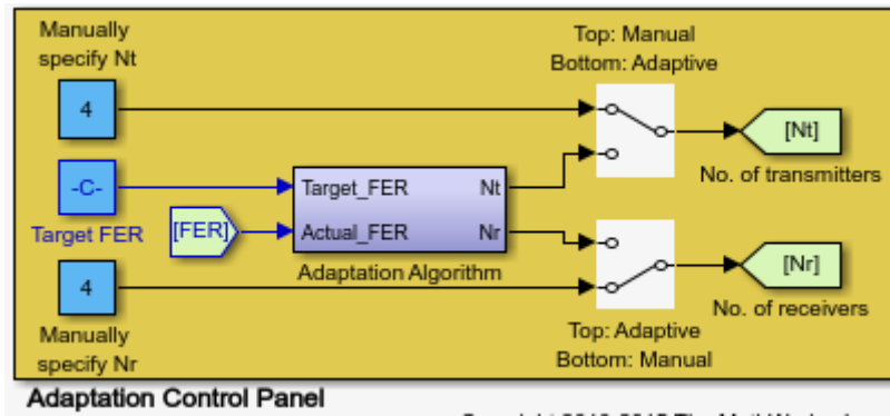
Рис. 4.55. Настройка блока Adaptation Control Panel для исследования случая ММО 4x4.
