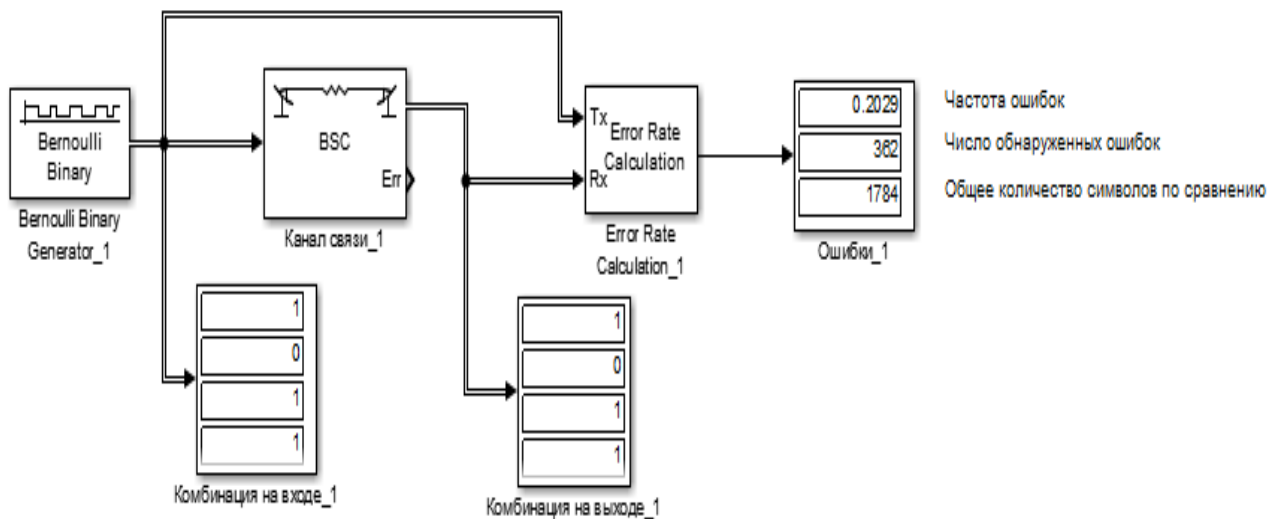
Рис. 3.46. Линия передачи без преобразований
