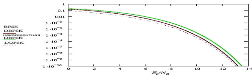
Рис. 1.18. Сравнение энергетической эффективности модуляций с относительным кодированием: DBPSK, DQPSK и некогерентной DBPSK.
