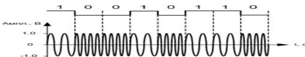
Рис. 1.23. Частотная манипуляция
