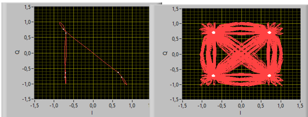
Рис. 1.65. Диаграмма QPSK. 10 символов в сообщении (слева), 1000 символов в сообщении (справа).
