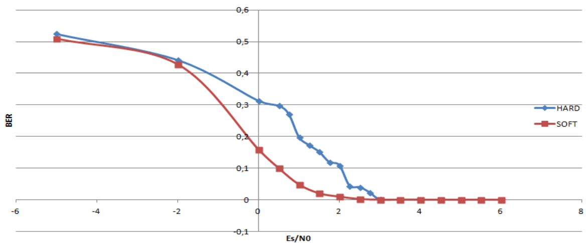
Рис. 3.95. График зависимости коэффициента битовых ошибок от отношения сигнал/шум для жесткого (синий) и мягкого (красный) принятий решений сверточного декодирования Витерби.
