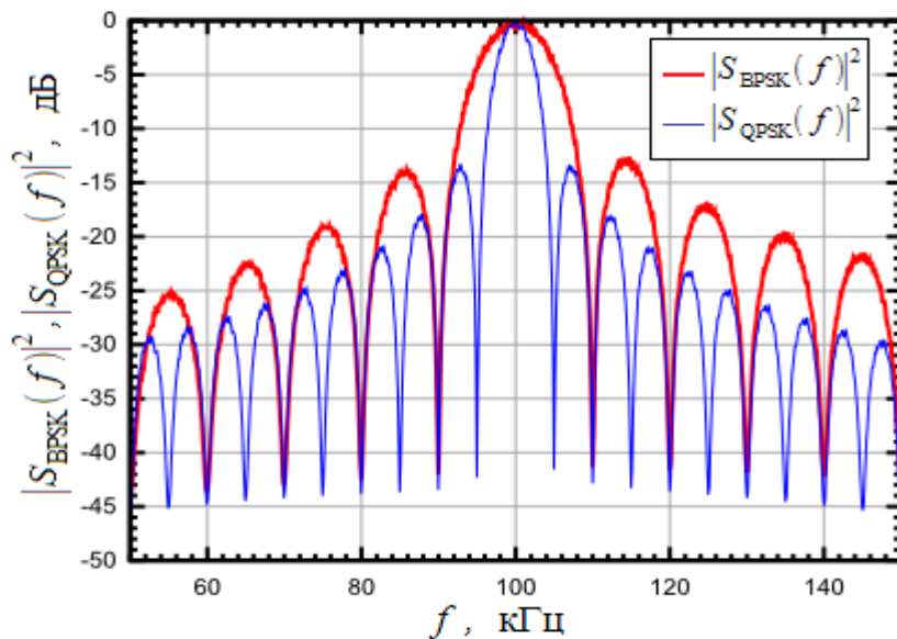
Рис. 1.58. Спектр QPSK сигнала.
