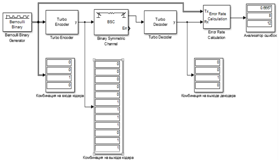
Рис. 3.116. Модель системы связи с использованием турбо-кодов
