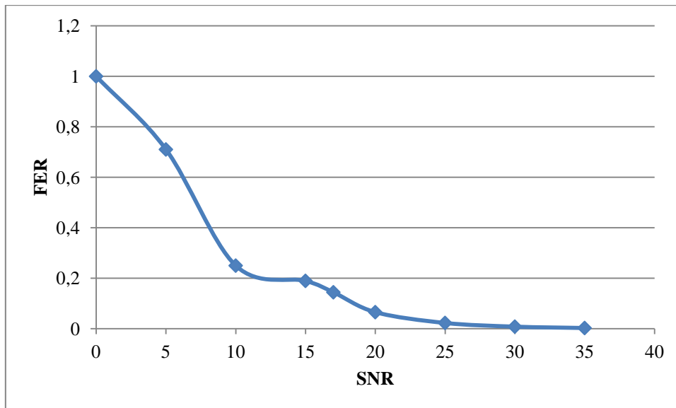
Рис. 4.57. Зависимости вероятности кадровой ошибки от отношения сигнал\шум для адаптивной модели ММО
