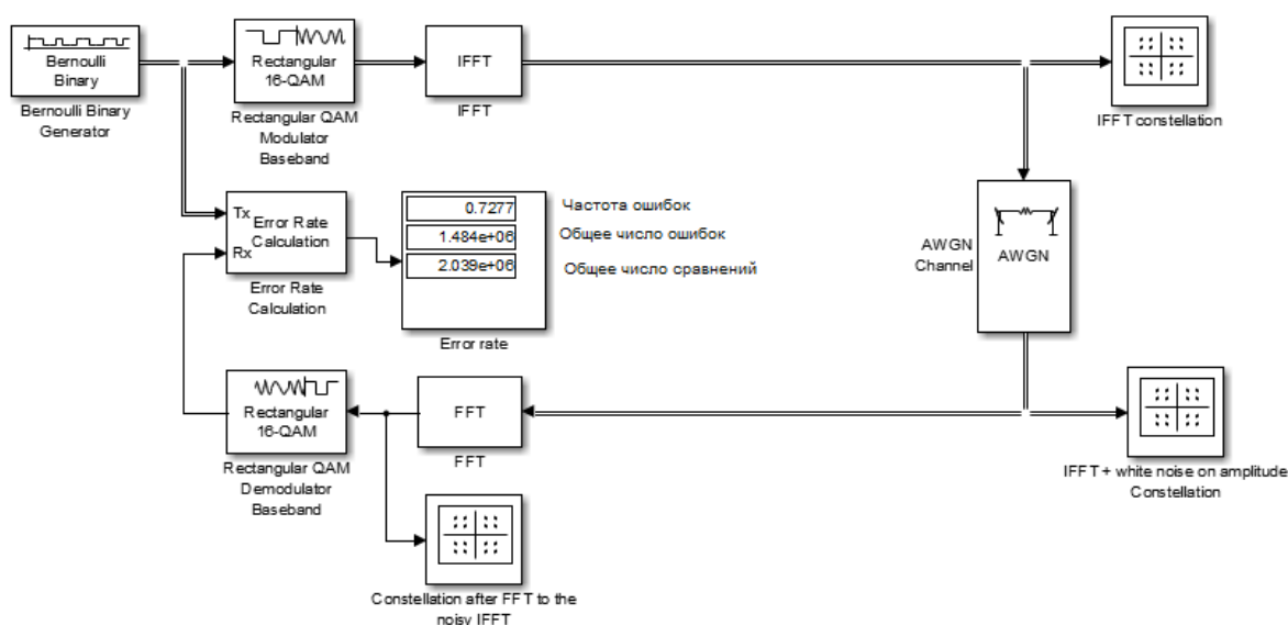
Рис. 4.41. Модель МАТЛАБ для исследования системы OFDM.
