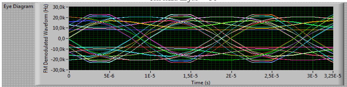
Рис. 1.44. Глазковая диаграмма сигнала с GMSK модуляцией при BT = 0.3 , сигнал/шум = 80
