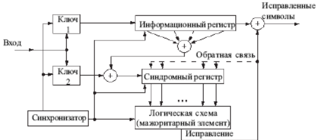
Рис. 5.11. Функциональная схема декодера Витерби кодера со скоростью 1/2.
