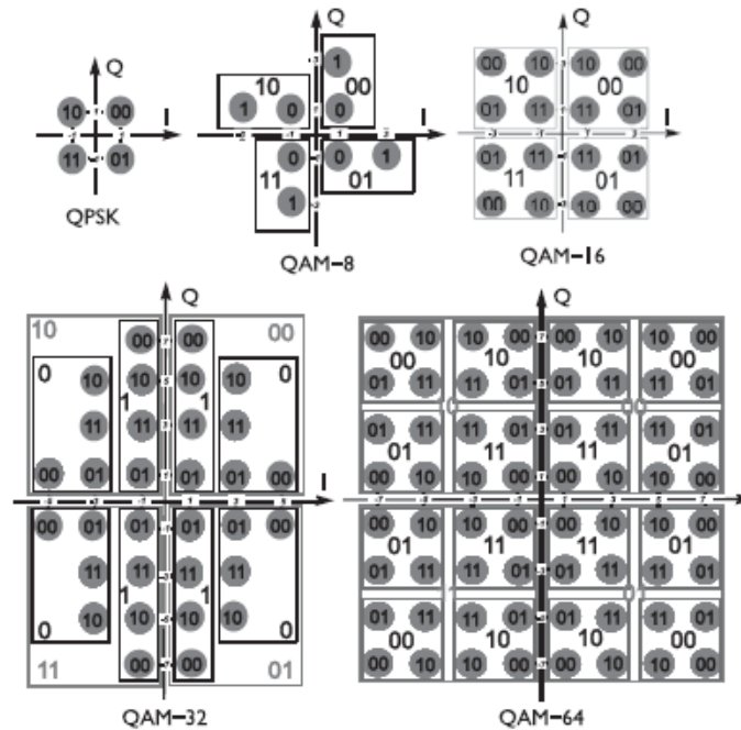
Рисю 4.32 - Варианты сигнальных созвездий: QPSK, QAM-8, QAM-16, QAM-32 и QAM-64.
