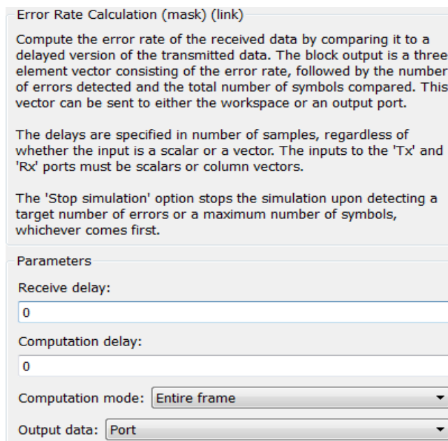
Рис. 3.13 Параметры Error Rate Calculation
