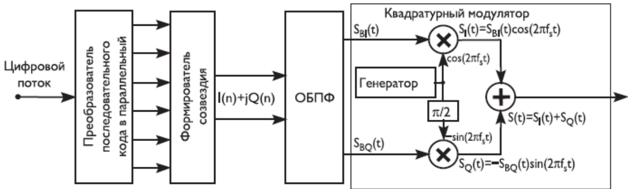
Рисунок 4.31 - Структурная схема идеального OFDM-модулятора.
