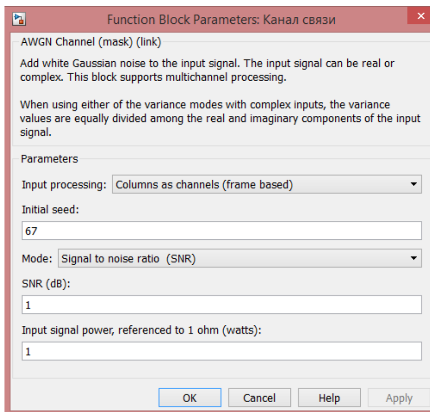
Рис. 3.61. Параметры блока «AWGN»
