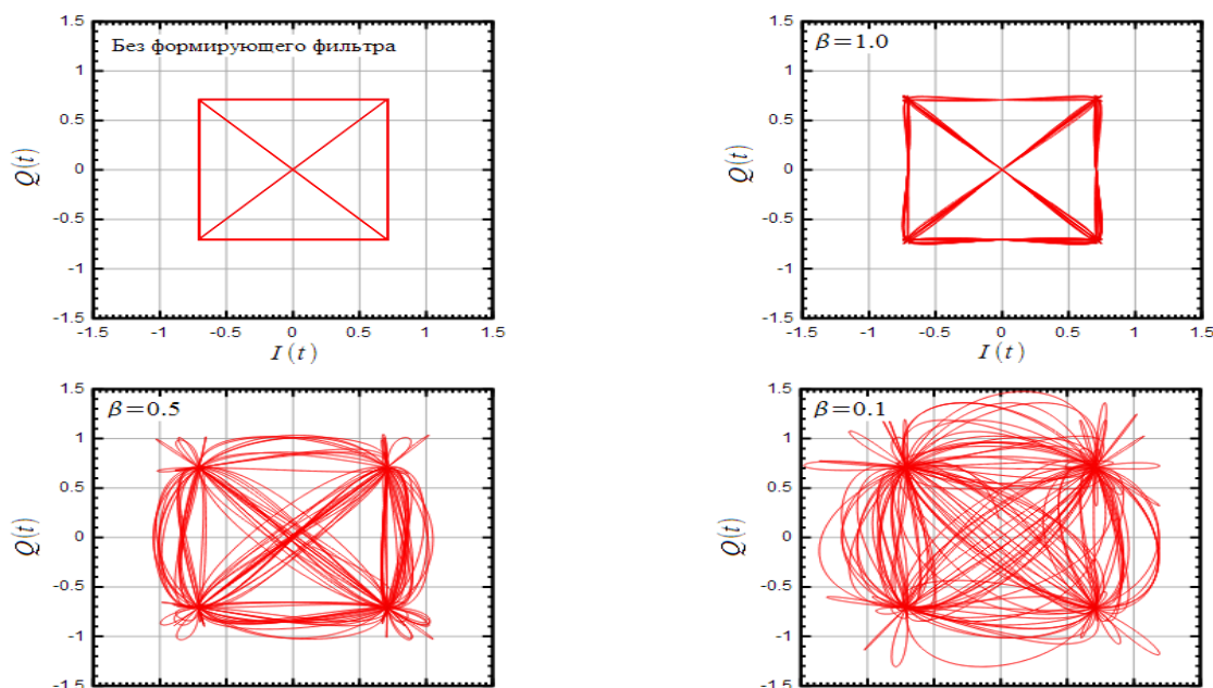
Рис. 1.62. Траектории движения вектора комплексной огибающей QPSK сигнала при различных параметрах формирующего фильтра Найквиста.
