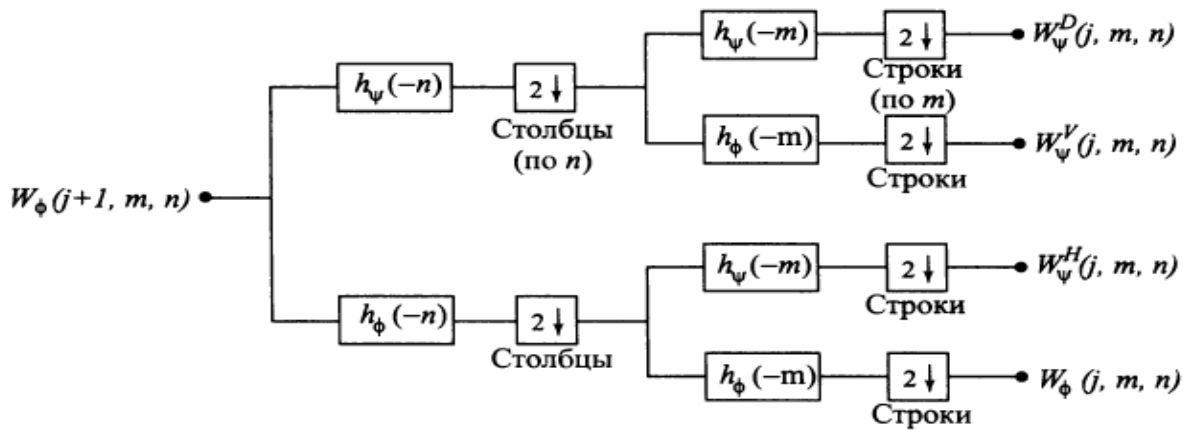
Рис. 2.53. Схема быстрого вейвлет-преобразования
