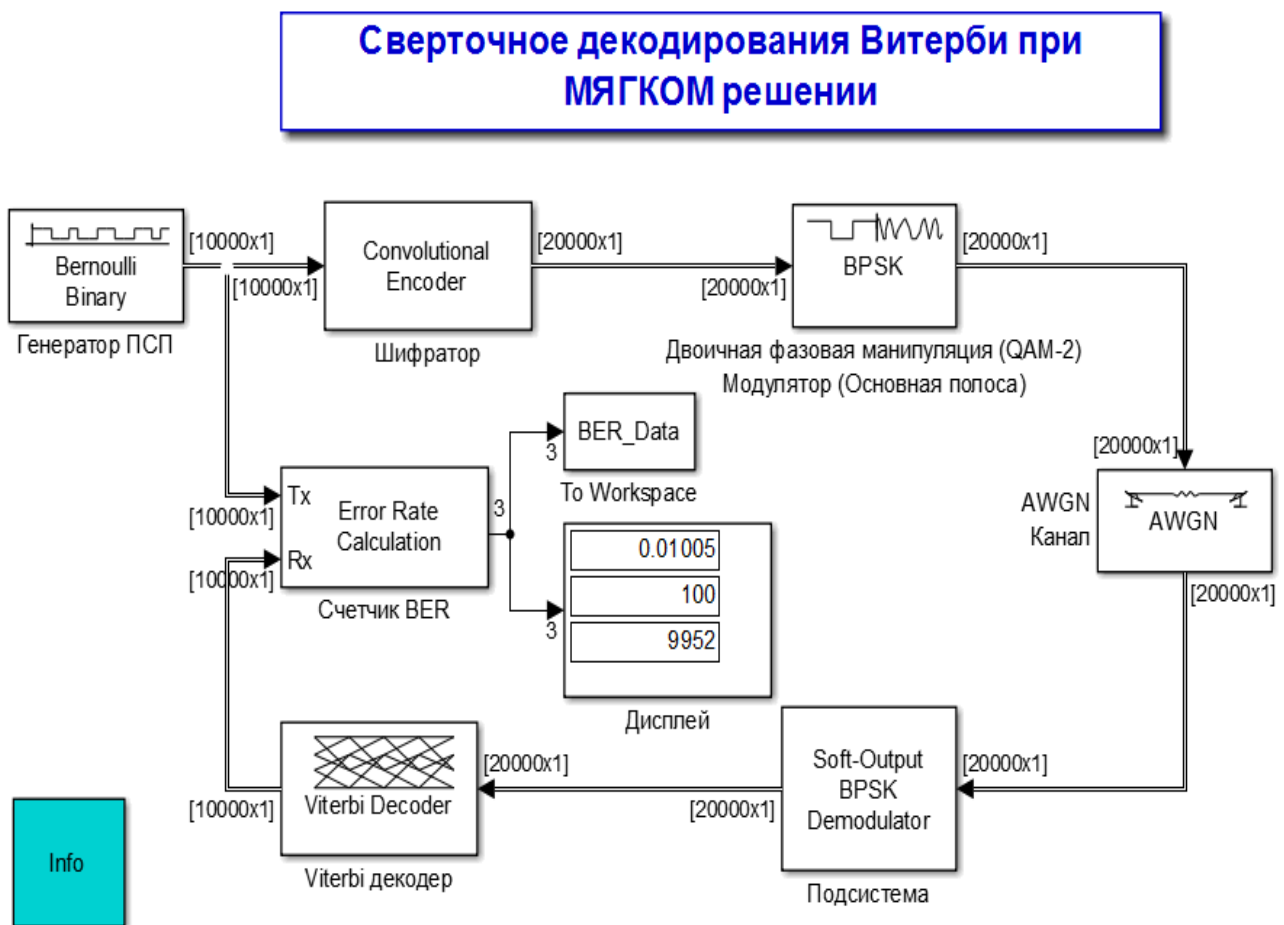
Рис. 3.93 – Модель сверточного декодера Витерби при «Мягком решении»
