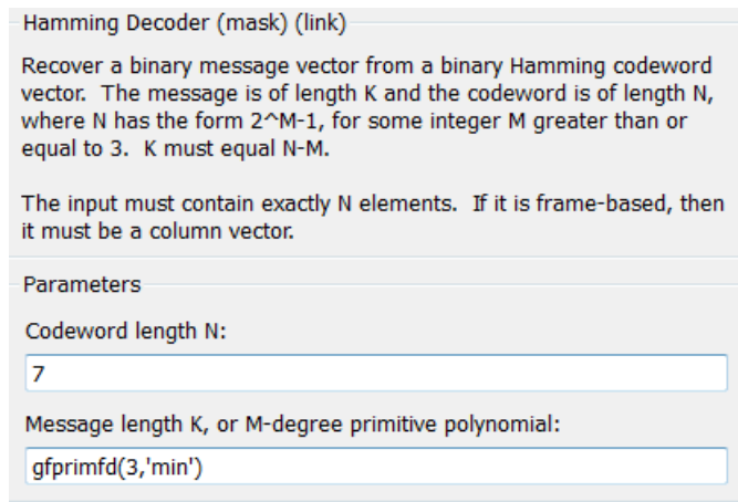
Рис. 3.12. Параметры Hamming Decoder
