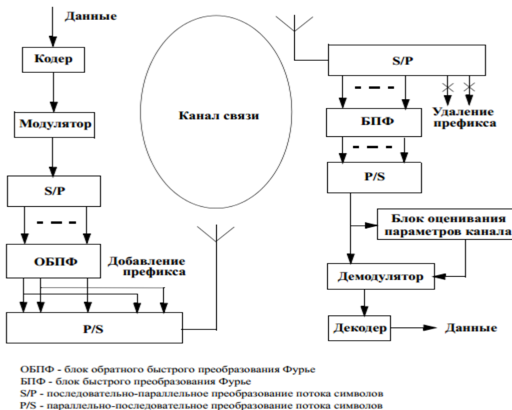
Рис. 4.24. Структурная схема системы связи с ортогональным частотным мультиплексированием
