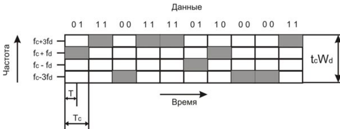
Рис. 1.24. Использование частоты схемой MFSK ( M = 4 )
