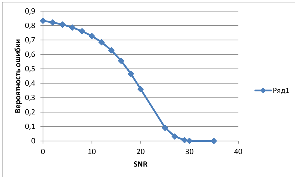
Рис. 4.49. Зависимость частоты ошибок от отношения сигнал/шум
