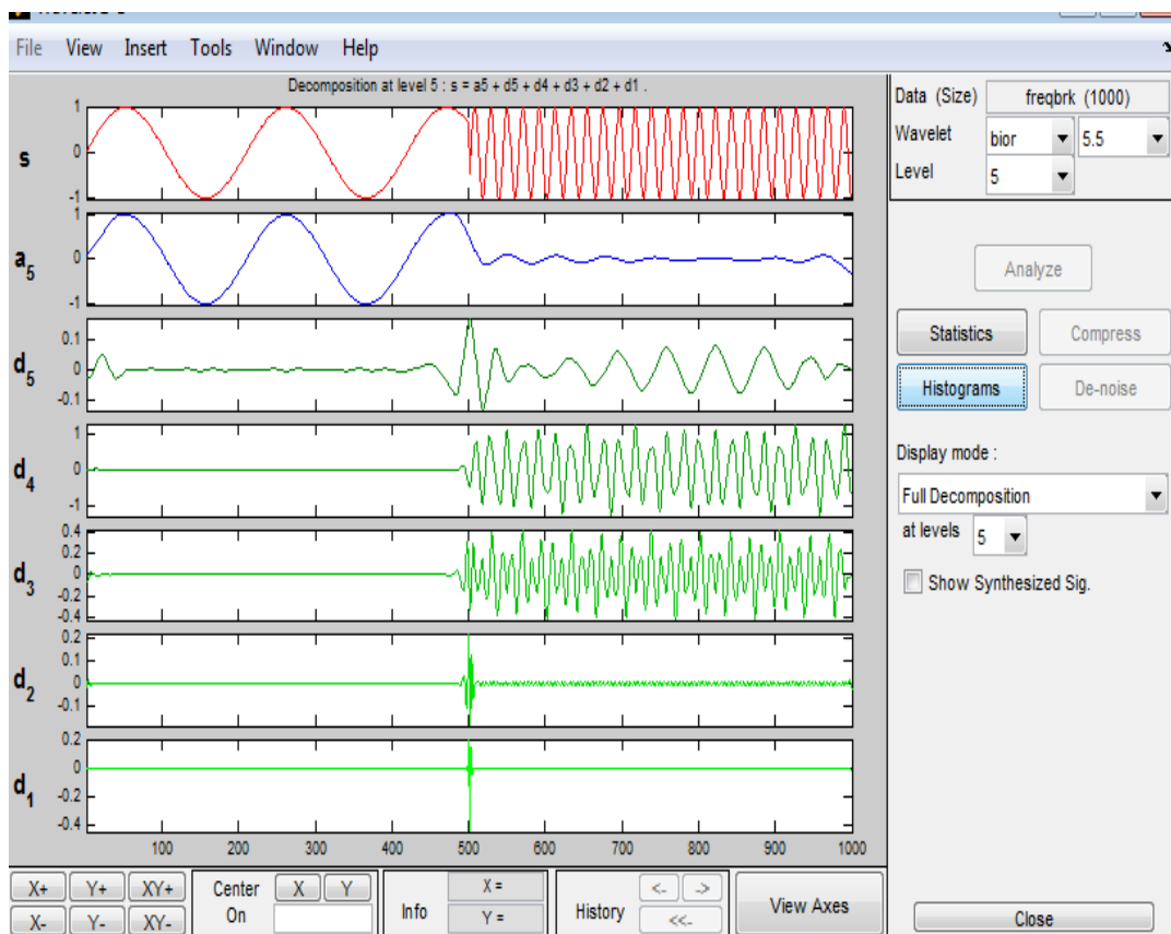
Рис. 2.70. Разложение сигнала при помощи биортогонального преобразования пятого уровня и порядка 5,5
