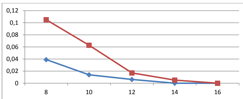
Рис. 1.32. Зависимость вероятности ошибки от отношения сигнал/шум
