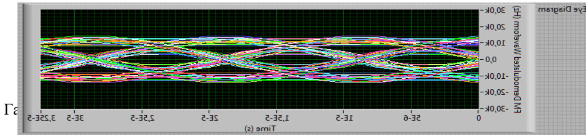
Рис. 1.43. Глазковая диаграмма сигнала с GMSK модуляцией при BT = 0.2 , сигнал/шум = 80
