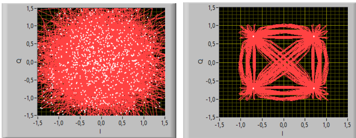
Рис. 1.66. Диаграмма QPSK. Отношение сигнал/шум 0 дБ (слева), Отношение сигнал/шум 60 дБ (справа).
