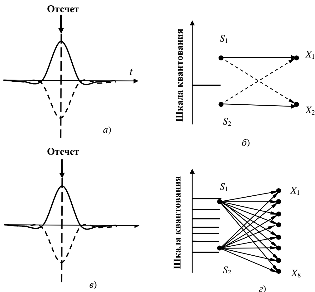
Рис. 3.91. Пояснение работы решающего устройства в демодуляторе
