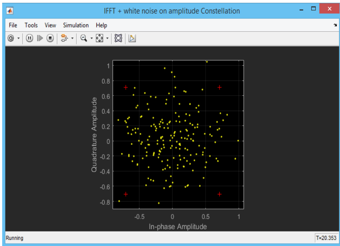
Рис. 4.50. Созвездие для значения отношения сигнал/шум 5 дБ.
