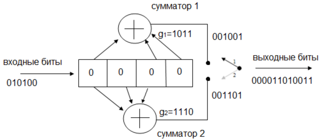
Рис. 3.85. Свёрточный кодер
