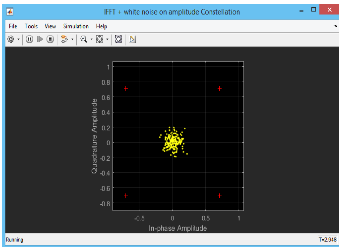
Рис. 4.52. Созвездие для значения отношения сигнал/шум 20 дБ.
