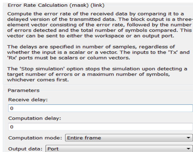
Рис. 3.49. ErrorRateCalculation (анализаторошибок)
