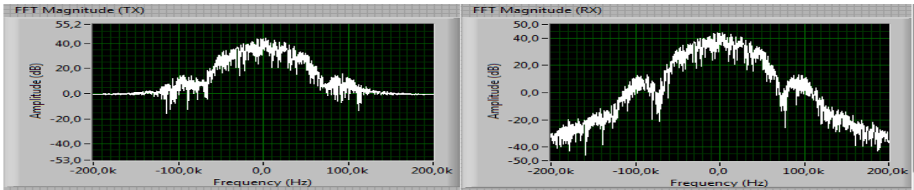
Рис. 1.41. Спектр передаваемого (слева) и принимаемого (справа) сигнала с GMSK модуляцией при BT = 0,3 , сигнал/шум = 80
