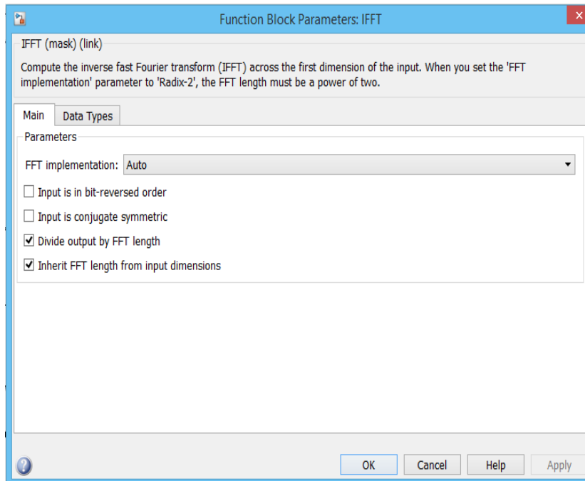
Рис. 4.44. Настройки блока преобразования Фурье
