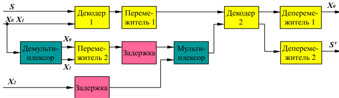
Рис. 3.141. Структурная схема одной итерации турбо-декодера при двухкаскадном кодировании
