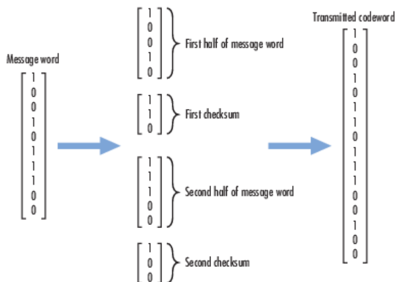
Рис. 3.55. Принцип работы кодера CRC
