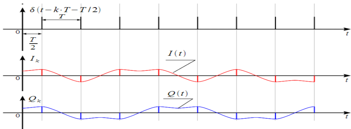
Рис. 1.61. Поясняющие графики.
