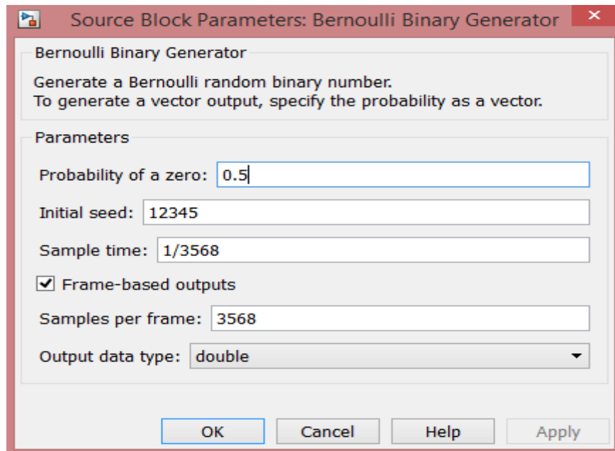
Рис. 3.144. Параметры блока «Bernoulli Binary Generator»
