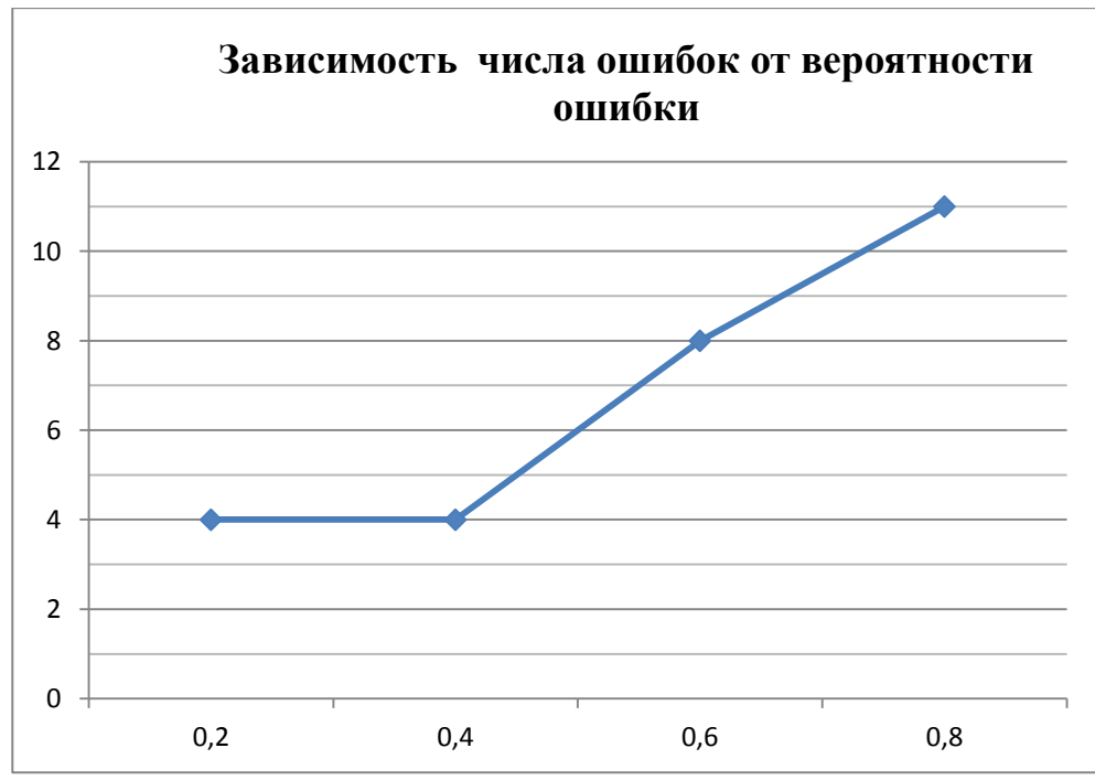
Рис. 3.23. График зависимости числа ошибок (OY) от вероятности ошибки (OX) для кода Хэмминга (15,11)
