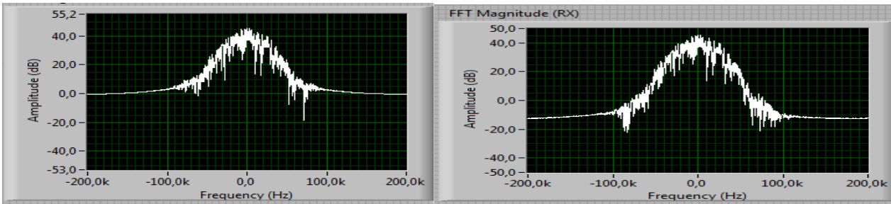
Рис. 1.40. Спектр передаваемого (слева) и принимаемого (справа) сигнала с GMSK модуляцией при BT = 0,2 , сигнал/шум = 80
