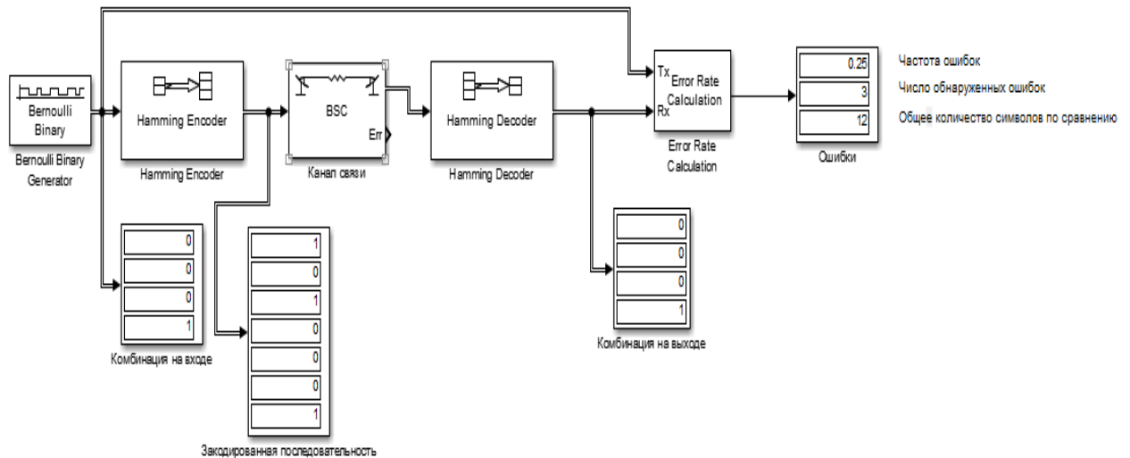
Рис. 3.8. Линия передачи с применением кода Хэмминга
