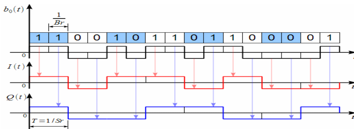
Рис. 1.53. Синфазная и квадратурная составляющие QPSK сигнала
