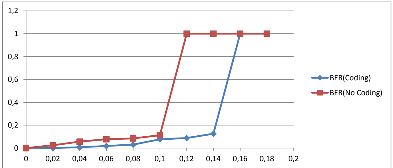
Рис. 3.122. График зависимости BER от Noise
