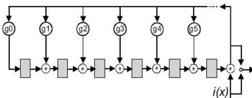
Рис. 3. 41. Схема кодировщика P-C
