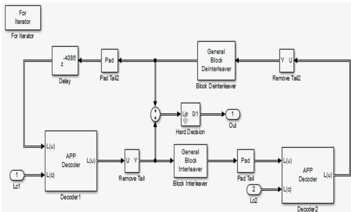
Рисунок 3.154. Схема турбо-декодера
