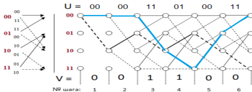
Рис. 3.87. Решетка декодера
