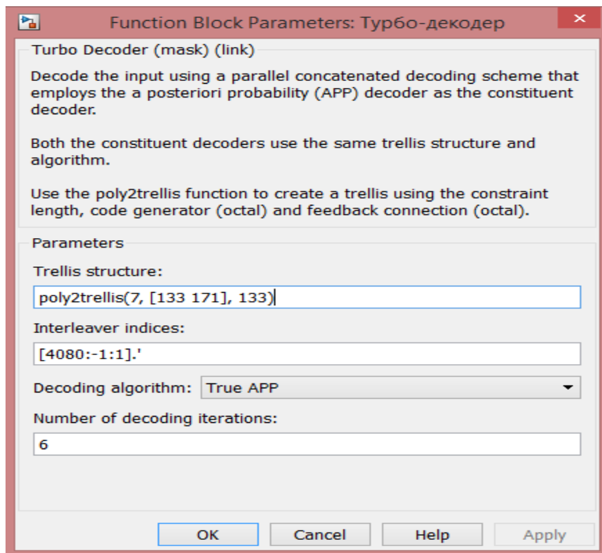
Рис. 3.152. Параметры блока «Turbo decoder»
