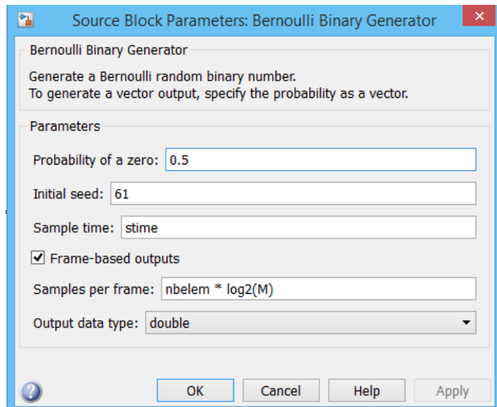
Рис. 4.42. Настройки блока генератора ПСП
