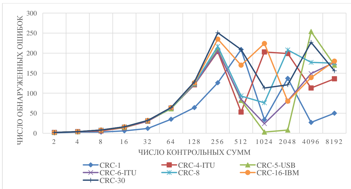
Рис. 3.63. График зависимости числа обнаруженных ошибок от числа контрольных сумм для различных полиномов CRC-кода
