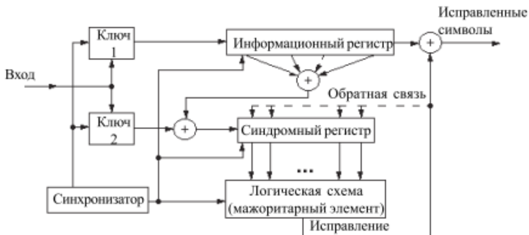
Рис. 3.70. Общая схема декодера для сверточного кода
