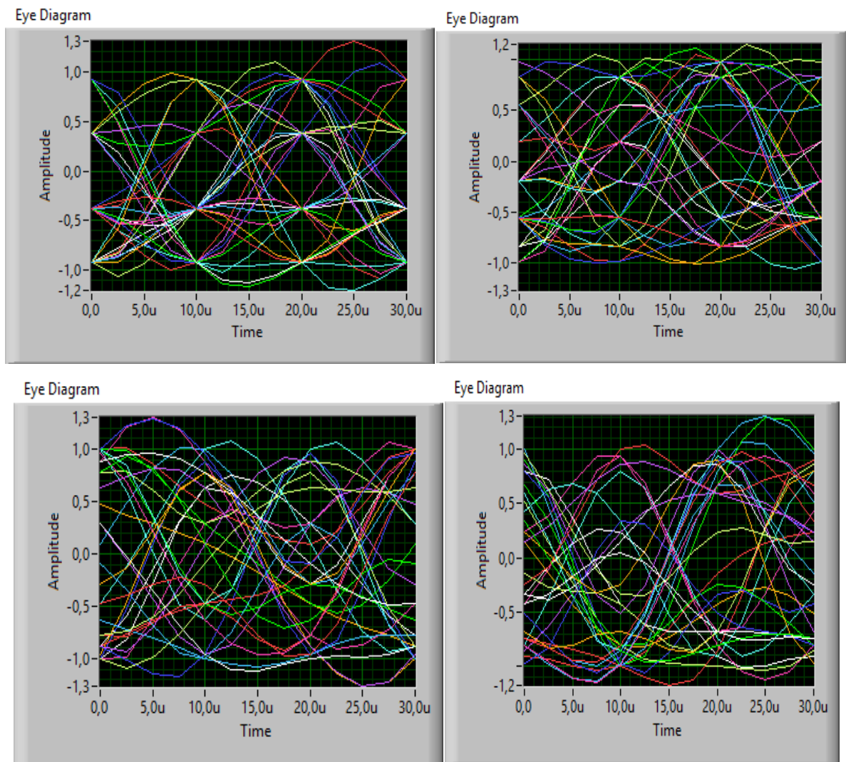
Рис. 1.70. Глазковые диаграммы для разных значений M на оси I (слева на право – сверху вниз): 2,4,8,16,32,64
