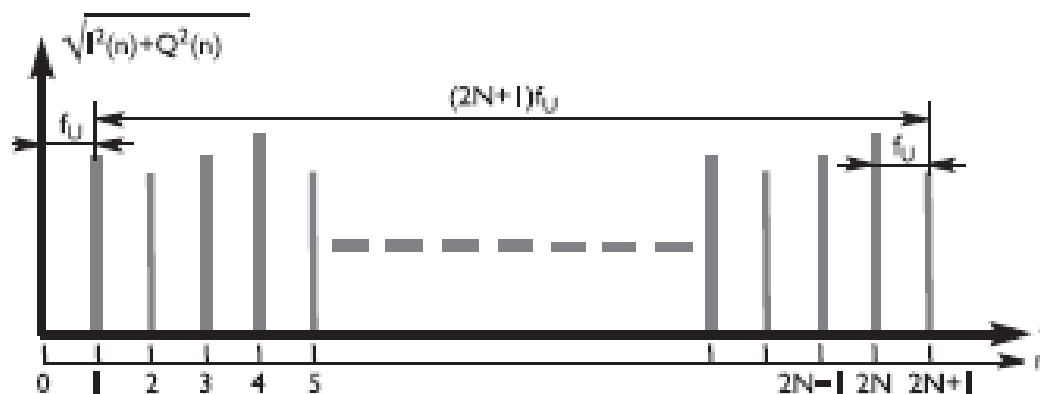
Рисунок 4.33 - График спектральных составляющих ОБПФ.
