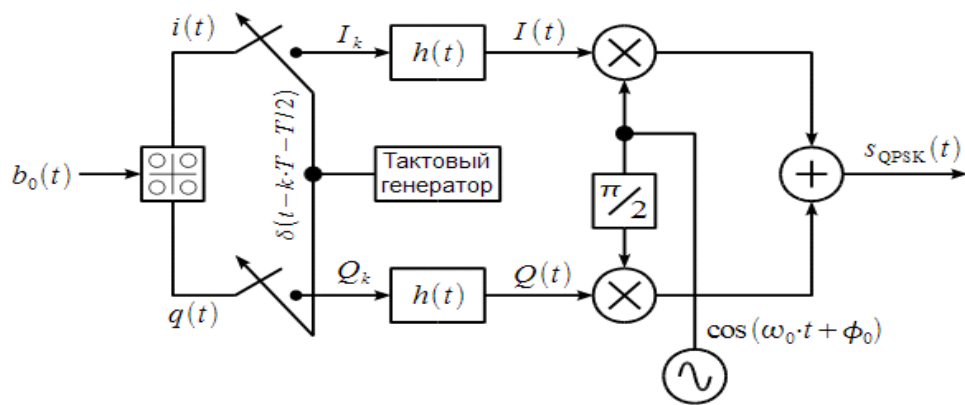
Рис. 1. 60. Структурная схема QPSK модулятора с использованием формирующего фильтра
