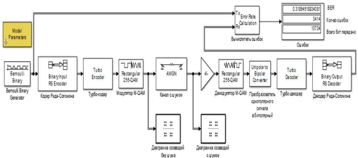
Рис. 3.143. Разработанная модель исследования каскадных кодов
