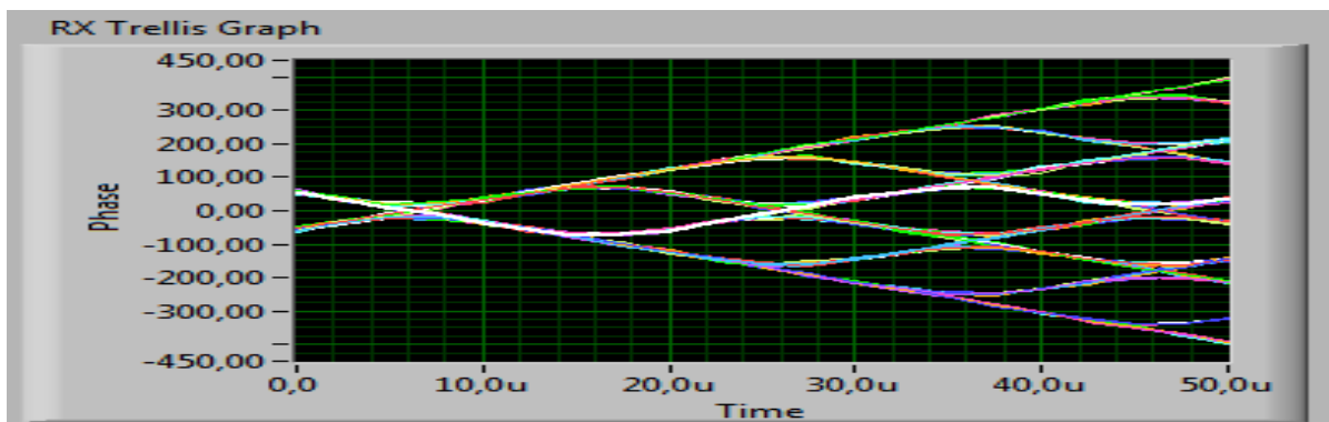
Рис. 1.48. Фазовая диаграмма полученного сигнала при BER= 10^{-4} , сигнал/шум = 28
