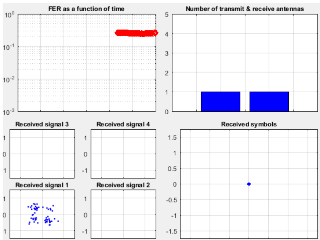
Рис. 4.58. Работа блока Signal Visualization (SISO)
