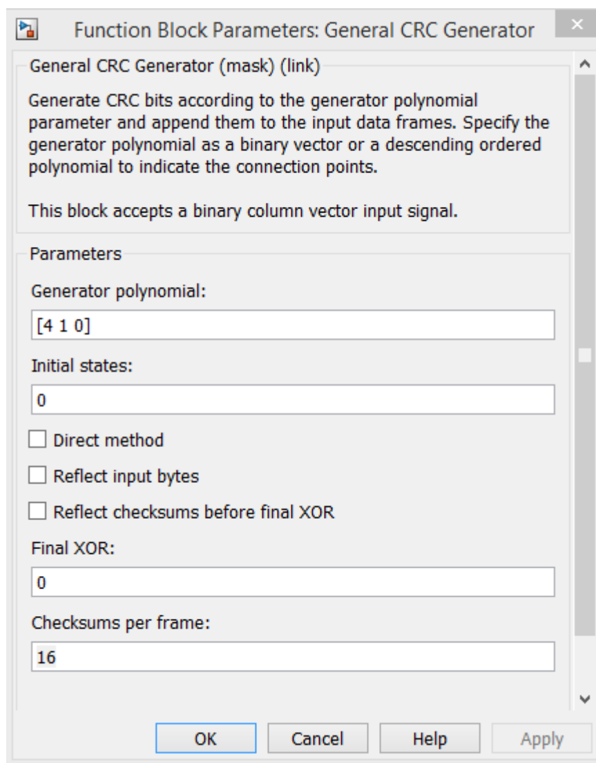
Рис. 3.60. Параметры блока «General CRC Generator»
