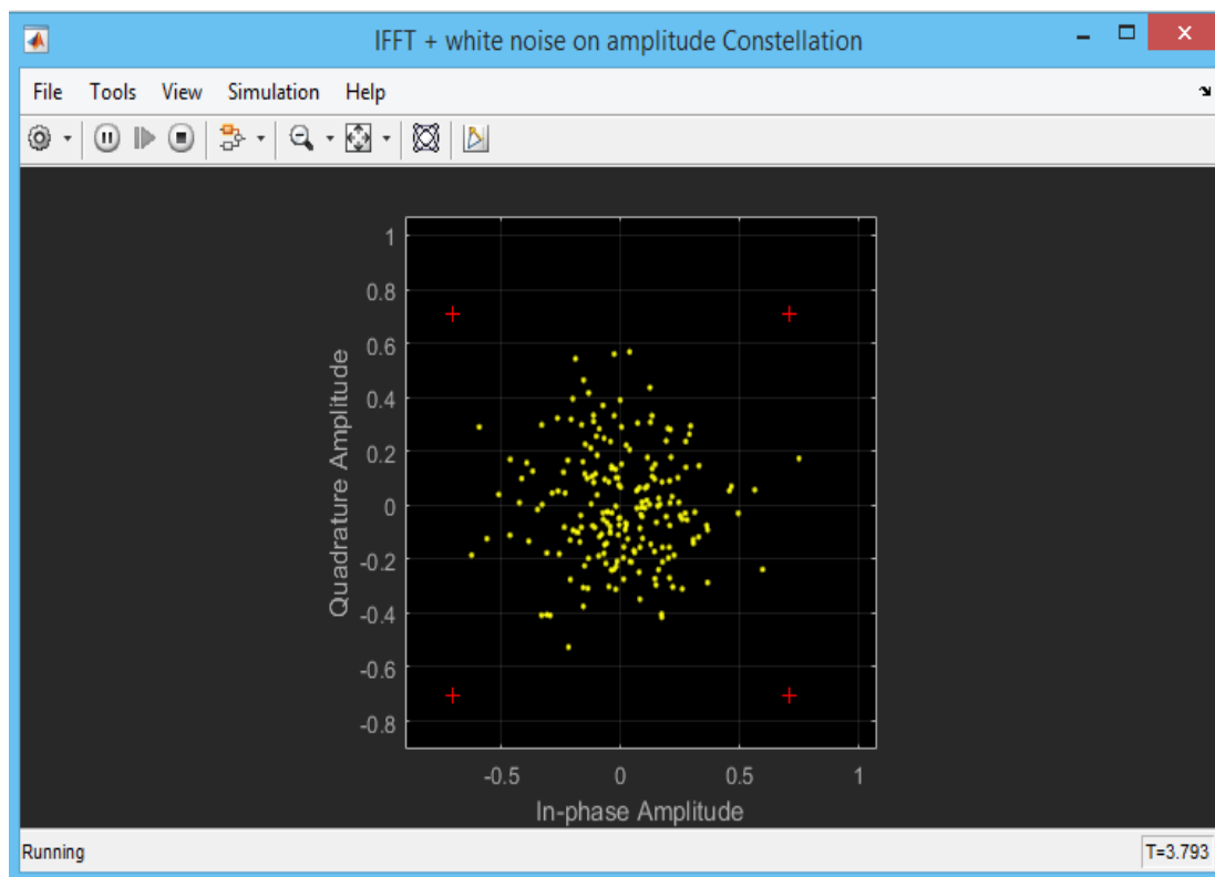
Рис. 4.51. Созвездие для значения отношения сигнал/шум 10 дБ.
