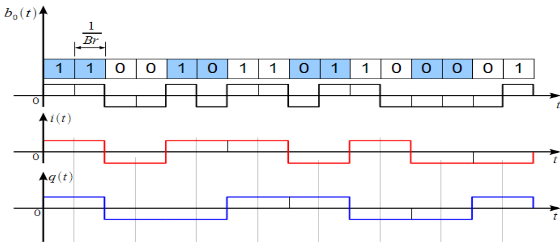
Рис. 1.61. Поясняющие графики.
