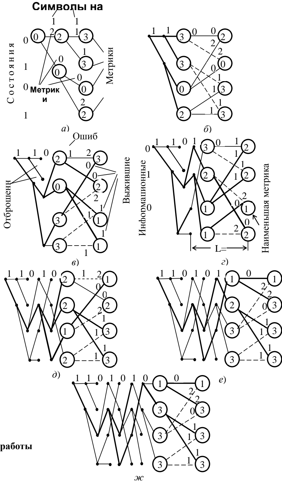
Рис. 3.92. Декодирование кода (7;5)
