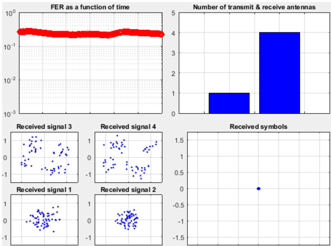
Рис. 4.58. Работа блока Signal Visualization (SIMO: 1 передатчик - 4 приёмник)
