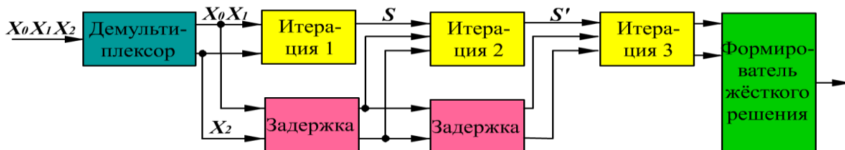
Рис. 3.142. Структурная схема трёх итерации турбо-декодера при двухкаскадном кодировании
