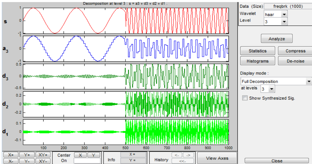
Рис. 2.58. Разложение сигнала
