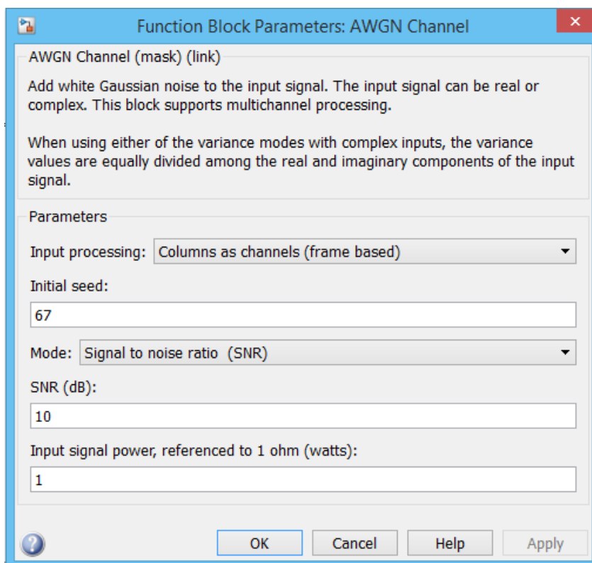
Рис. 4.45. Настройки блока канала с шумами
