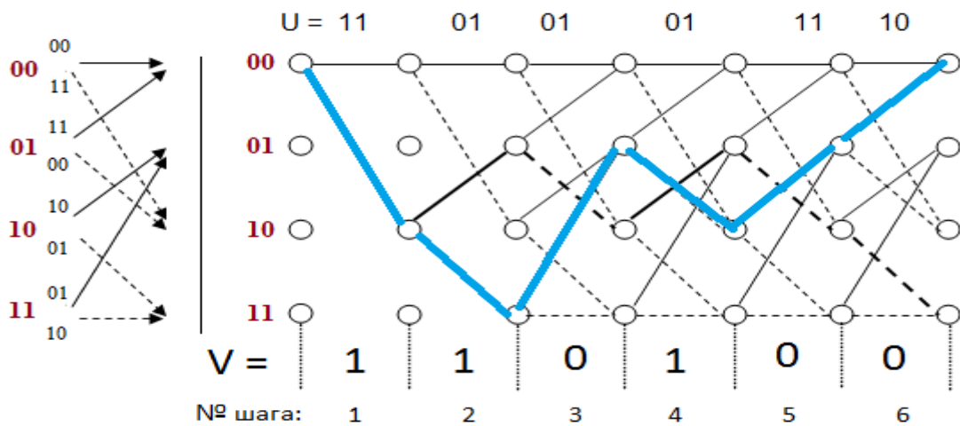
Рис. 3.84. Решетка декодера
