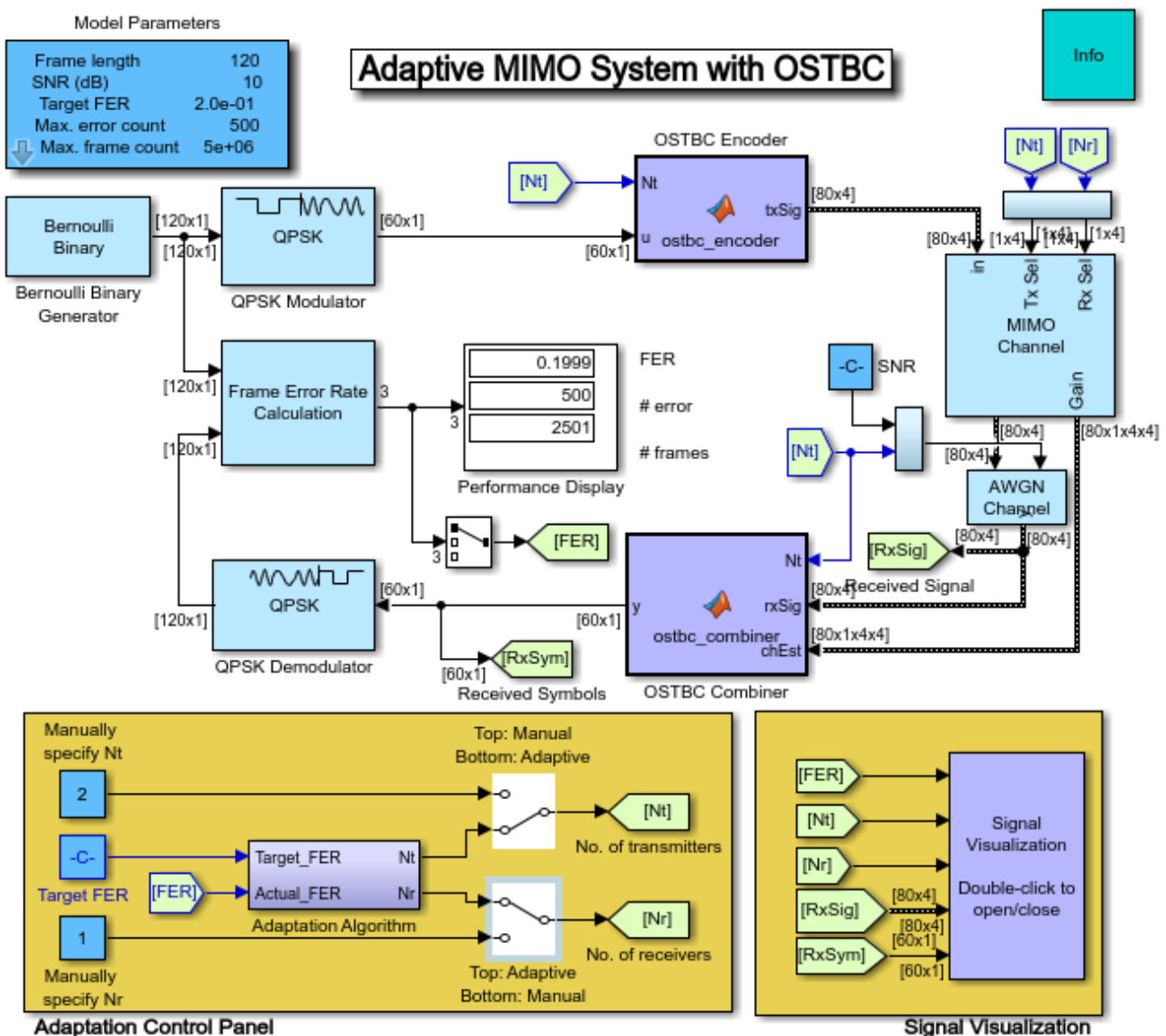
Рис. 4.54. Схема для исследования ММО.
