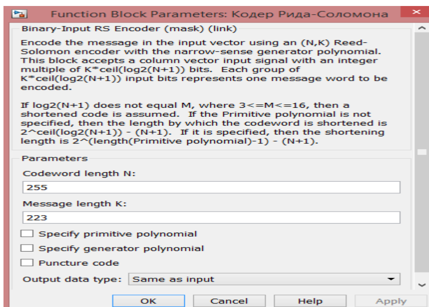
Рис. 3.145. Параметры блока «Binary Input RS Encoder»
