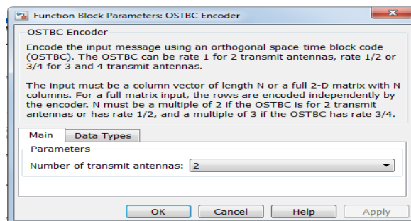
Рис. 4.12. Параметры блока: OSTBC Encoder
