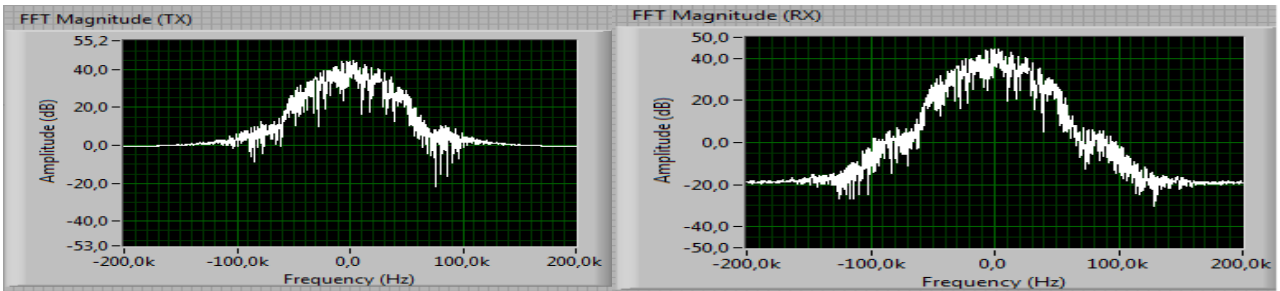
Рис. 1.41. Спектр передаваемого (слева) и принимаемого (справа) сигнала с GMSK модуляцией при BT = 0,3 , сигнал/шум = 80
