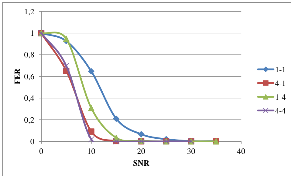
Рис. 4.61. Зависимости вероятности кадровой ошибки от SNR
