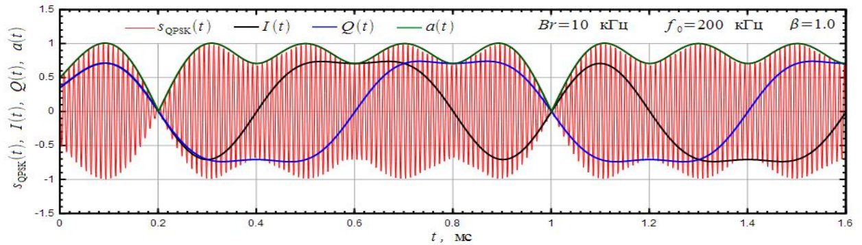
Рис. 1.63. Осциллограмма QPSK сигнала при использовании формирующего фильтра Найквиста
