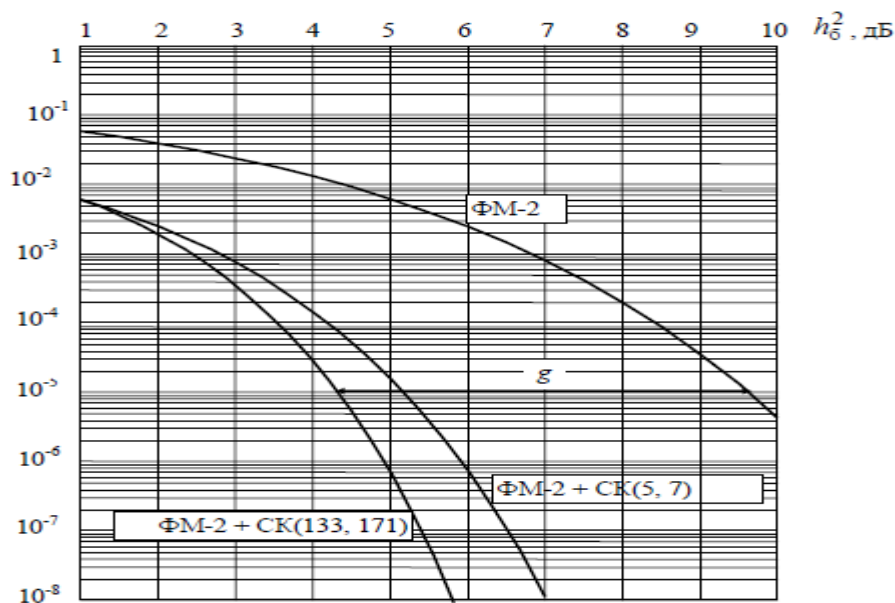
Рис. 5.2. Помехоустойчивость декодирования сверточных кодов
