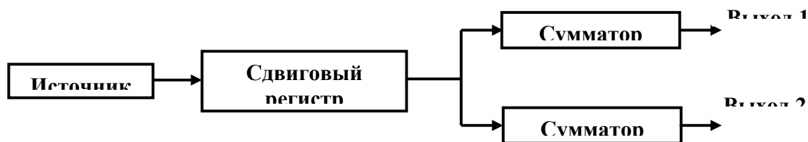
Рис. 5.3. Структурная схема сверточного кодера
