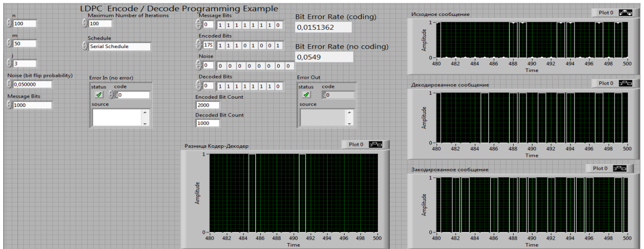
Рис.3.123. Панель управления аппаратно-программного комплекса LDPC кодера-декодера
