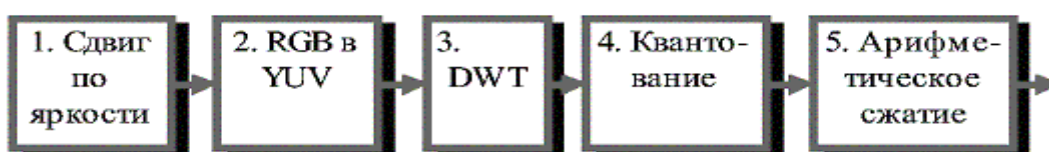
Рис. 2.76. Конвейер операций, используемый в алгоритме JPEG-2000
