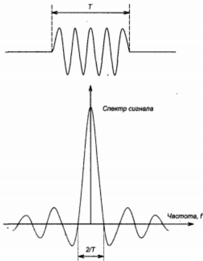
Рис. 4.25. Символ длительностью T и его спектральное представление
