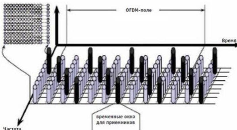
Рис. 4.30 - Маркеры синхронизации.
