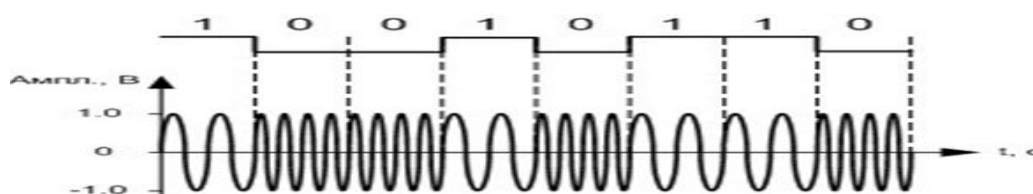
Рис. 1.23. Частотная манипуляция
