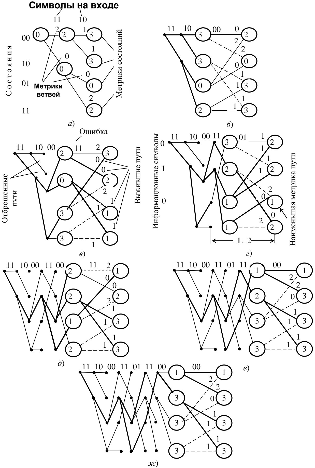
Рис. 3 – Декодирование кода (7;5)
