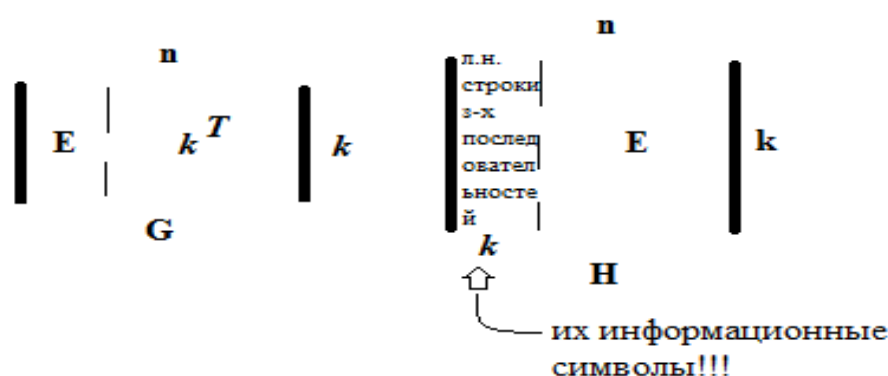
Рис. 3.3. Генераторная и проверочная матрицы
