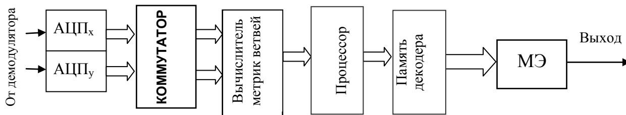
Рис. 4 – Структурная схема декодера Витерби
