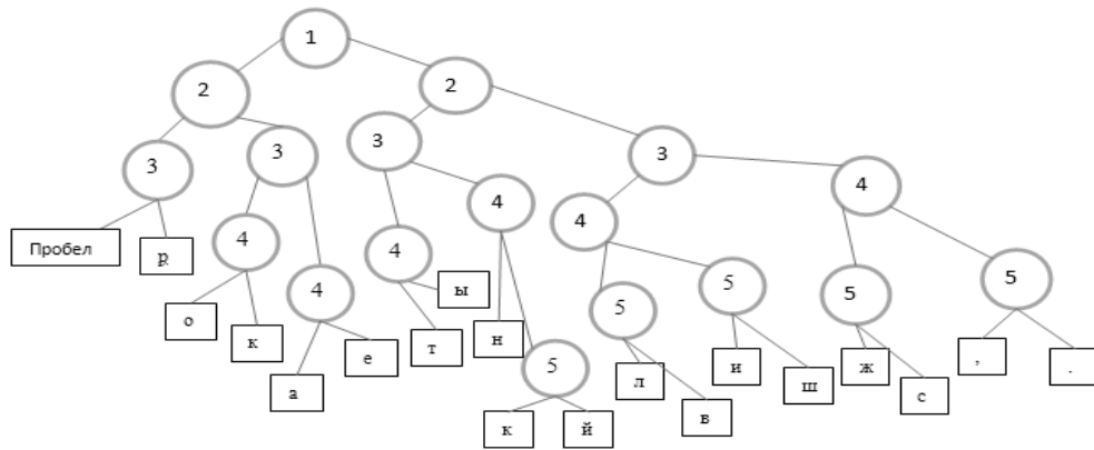
Рис.2.1. Результирующее дерево
