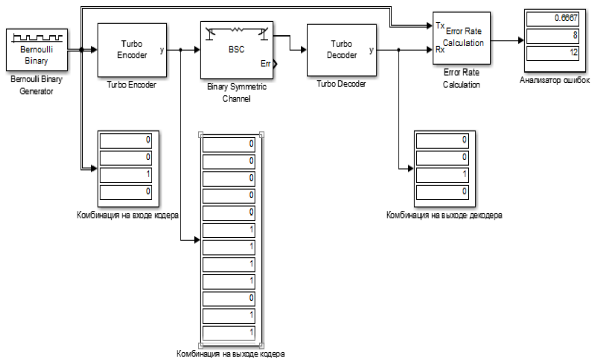
Рис. 3.116. Модель системы связи с использованием турбо-кодов
