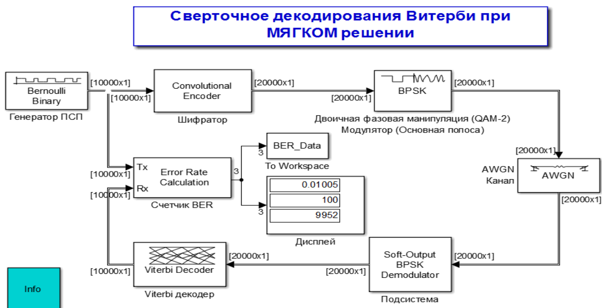
Рис. 5 – Модель сверточного декодера Витерби при «Мягком решении»
