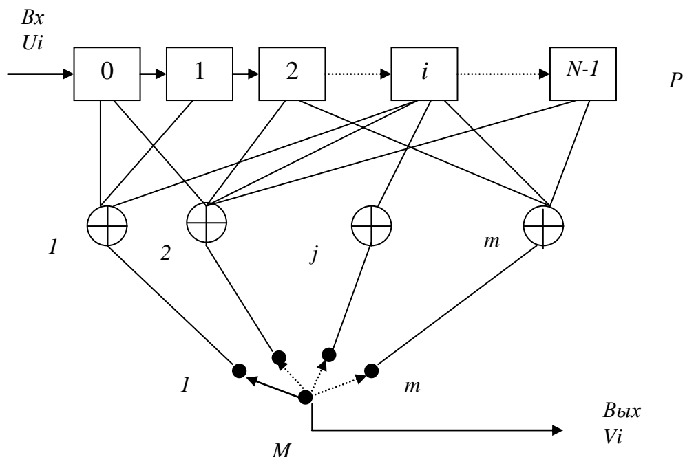
Рисунок 1 – Кодирующее устройство сверточного кода в общем виде
