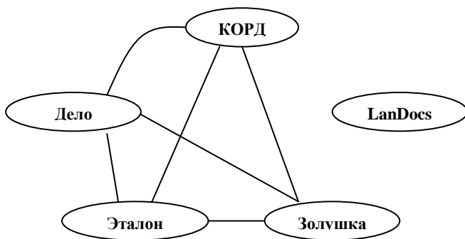
Рис. 2.1. Граф подобия
