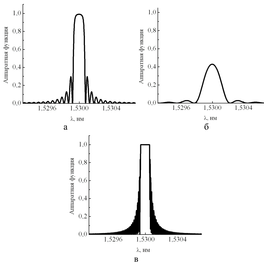
Рис. 2.21 — Аппаратные функции тонкопленочных фильтров, рассчитанных при различных значениях L : а — 1,5; б — 5,725; в — 20 мкм
