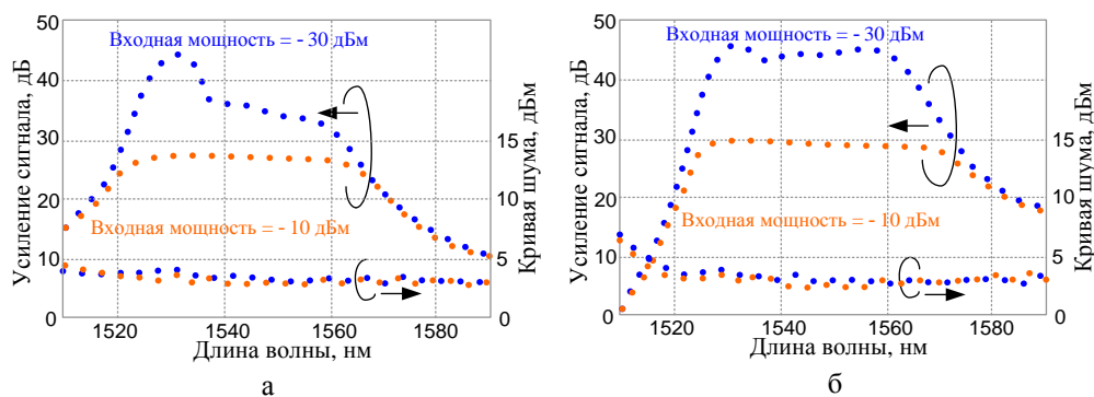
Рис. 2.11. — Зависимость коэффициента усиления (а) и коэффициента шума от длины волны для предусилителя (б) диапазона С
