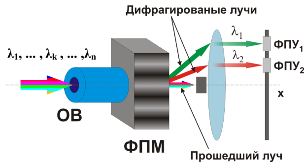
Рис. 2.31 — Применение наложенных голографических решеток в ФПМ для демультиплексирования группового оптического сигнала
