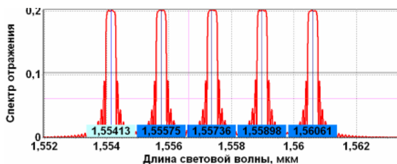
Рис. 4.7 — Область построения зависимости аппаратной функции
