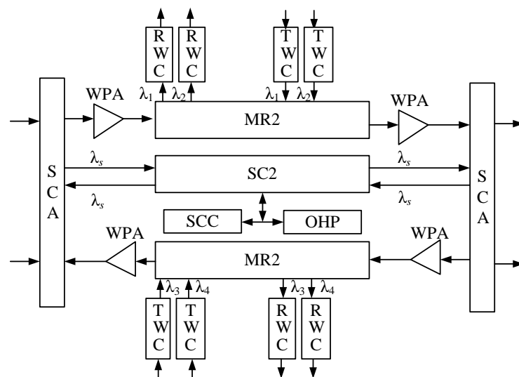
Рис. 1.14 — Структура OADM OptiX BWS 320G: MR2 — блок мультиплексирования ввода/вывода 2-х каналов; WPA — WDM — блок предварительного усилителя; WBA — WDM — блок усилителя-бустера; TWC — STM-16 — передающий блок преобразования длины волны; RWC — STM-16 — принимающий блок преобразования длины волны
