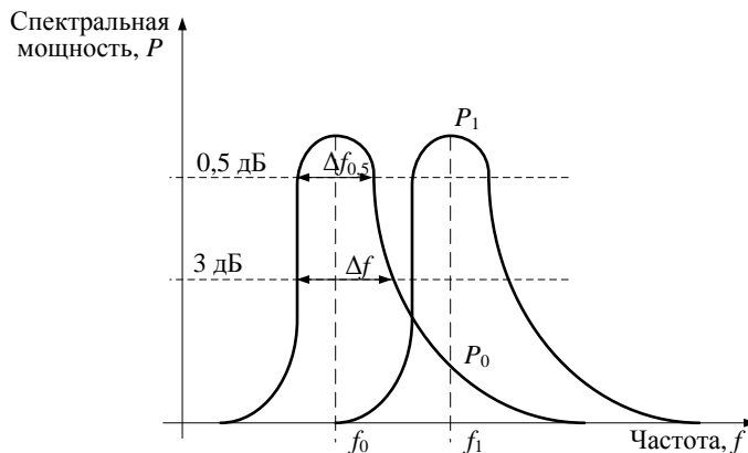
Рис. 1.21 — Частотная зависимость спектральной мощности
