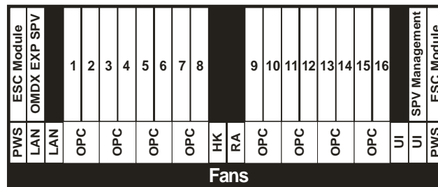
Рис. 2.25 — Конфигурация стойки
