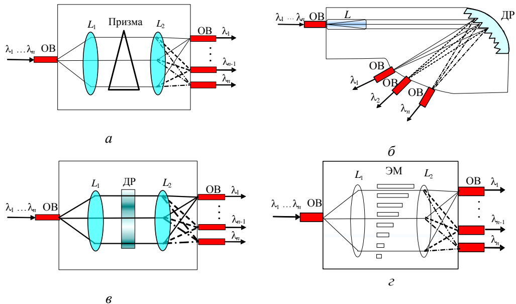
Рис. 1.18 — Схемы планарных интегрально-оптических волноводных структур на основе: а — призмы; б — отражательной дифракционной решетки; в — дифракционной решетки пропускающего типа; г — эшелона Майкельсона
