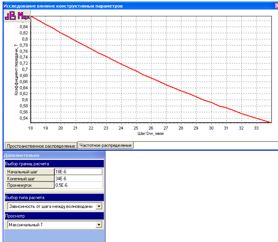
Рис. 4.28 — Вид окна «Исследование зависимости от параметров»
