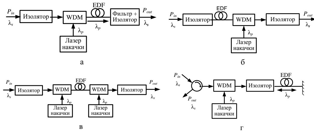
Рис. 2.2 — Основные схемы построения EDFA: а — прямая накачка; б — обратная накачка; в — двунаправленная накачка; г — отражательная накачка
