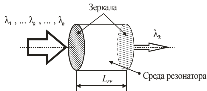
Рис. 2.26 — Конструкция фильтра на основе резонатора Фабри — Перро: L — длина резонатора
