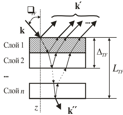
Рис. 2.19 — Брегговское отражение
