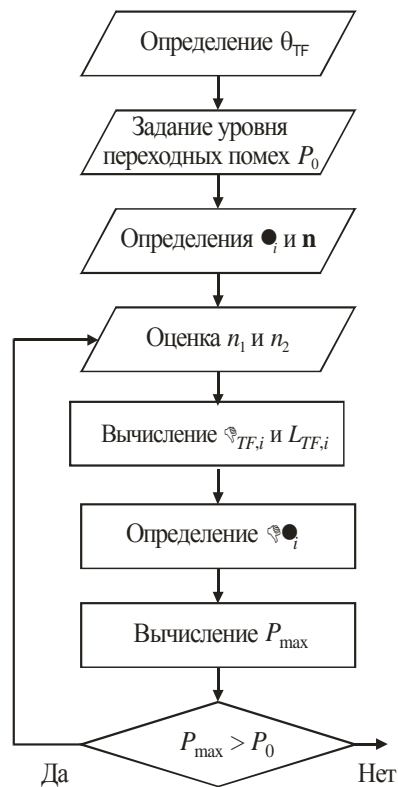
Рис. 2.22 — Блок-схема построения демультиплексора на основе интерференционных фильтров
