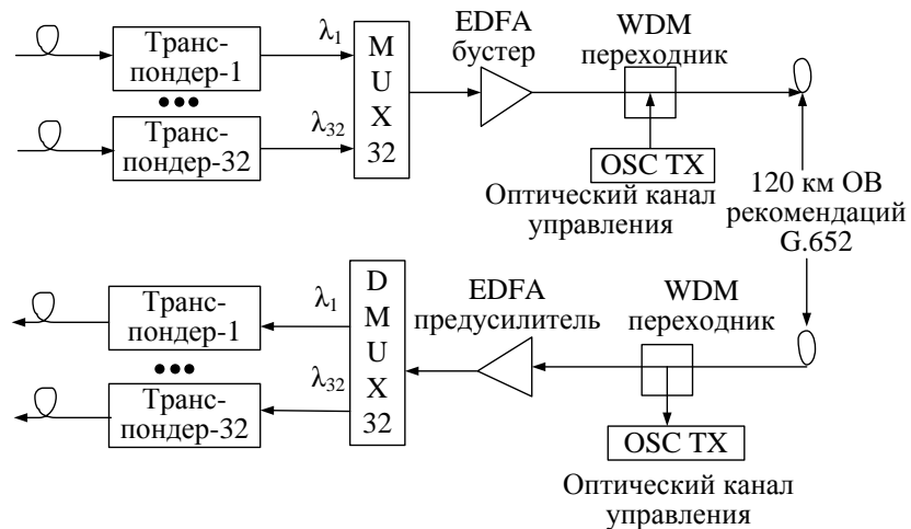
Рис. 1.13 — Структура OTM OptiX BWS 320G
