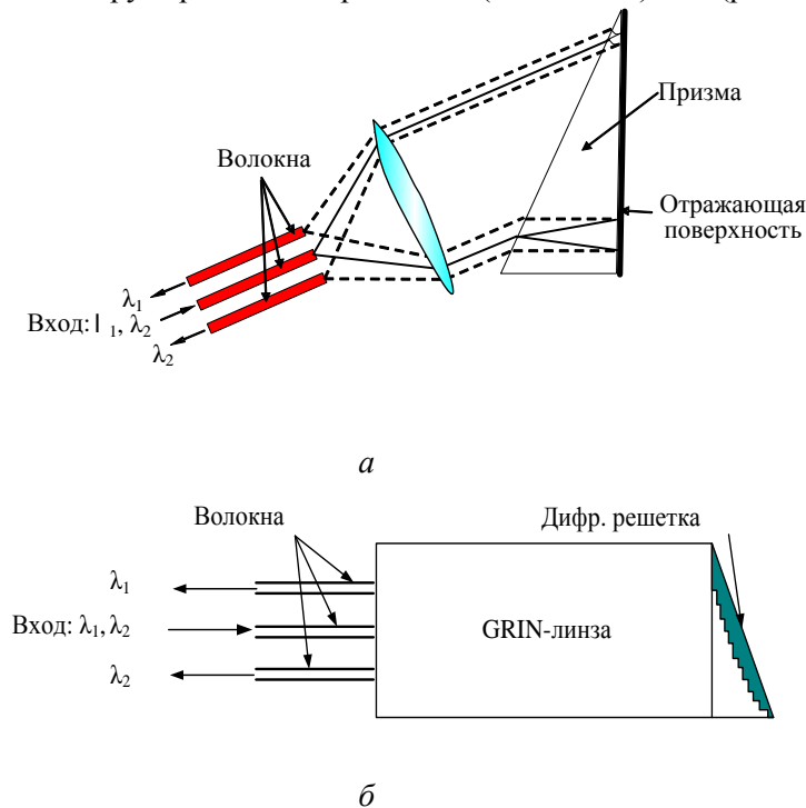
Рис. 1.16. Схема демultipлексора WDM: а — на отражающей призме; б — на отражающей плоской решетке
