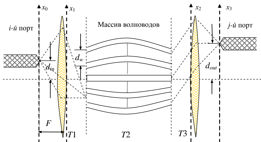
Рис. 2.39 — Оптическая схема AWG
