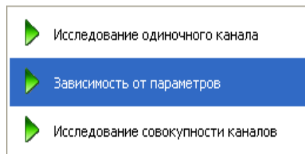
Рис. 4.26 — Окно «Параметры»
