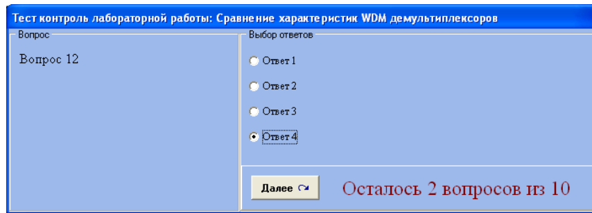
Рис. 4.22 — Окно тест-контроля
