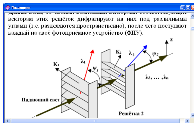
Рис. 4.21 — Информационное окно
