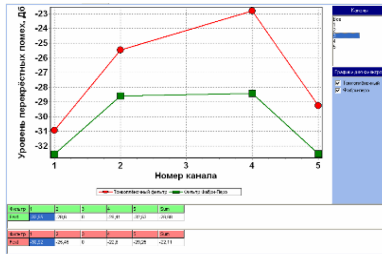
Рис. 4.13 — Информационное окно
