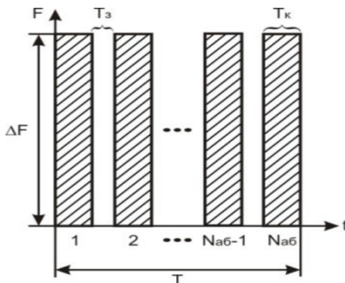
Рис. 1.4.2. Принцип временного разделения каналов
