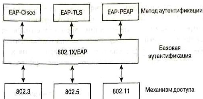
Рис. 1.6.2. Стандарт 802.1X и топологии канального уровня.
