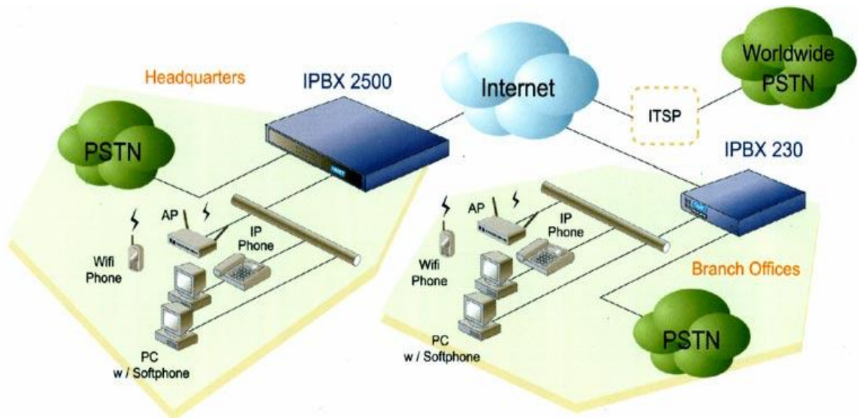
Рис. 8. Пример применения IPBX 2500 и IPBX 230
