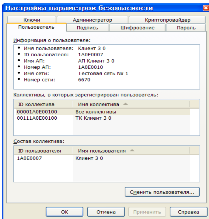
Рис. 77.Окно Настройка параметров безопасности
