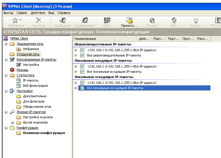
Рис. 78. Фильтры открытой сети
