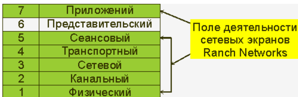
Рис. 17. Обеспечение функций безопасности на уровнях модели OSI
