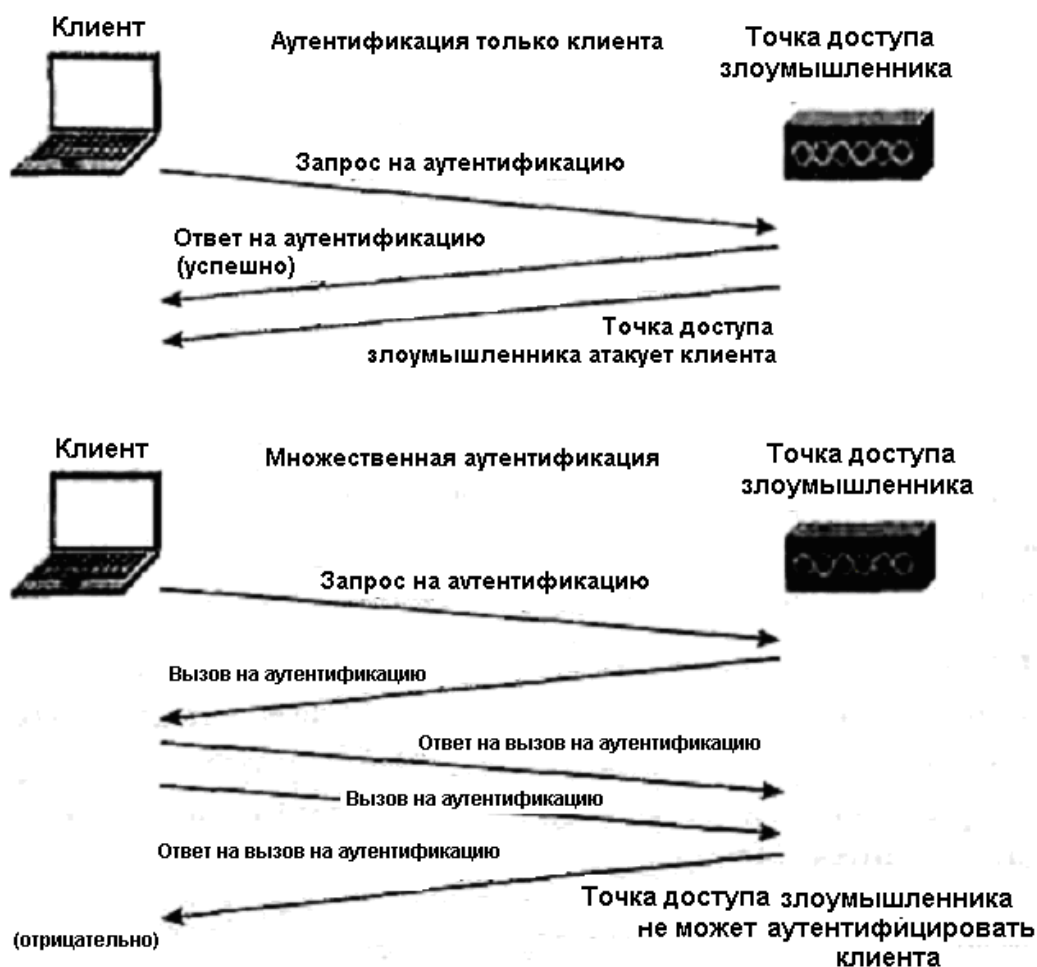
Рис. 1.6.1. Односторонняя и взаимная аутентификация.
