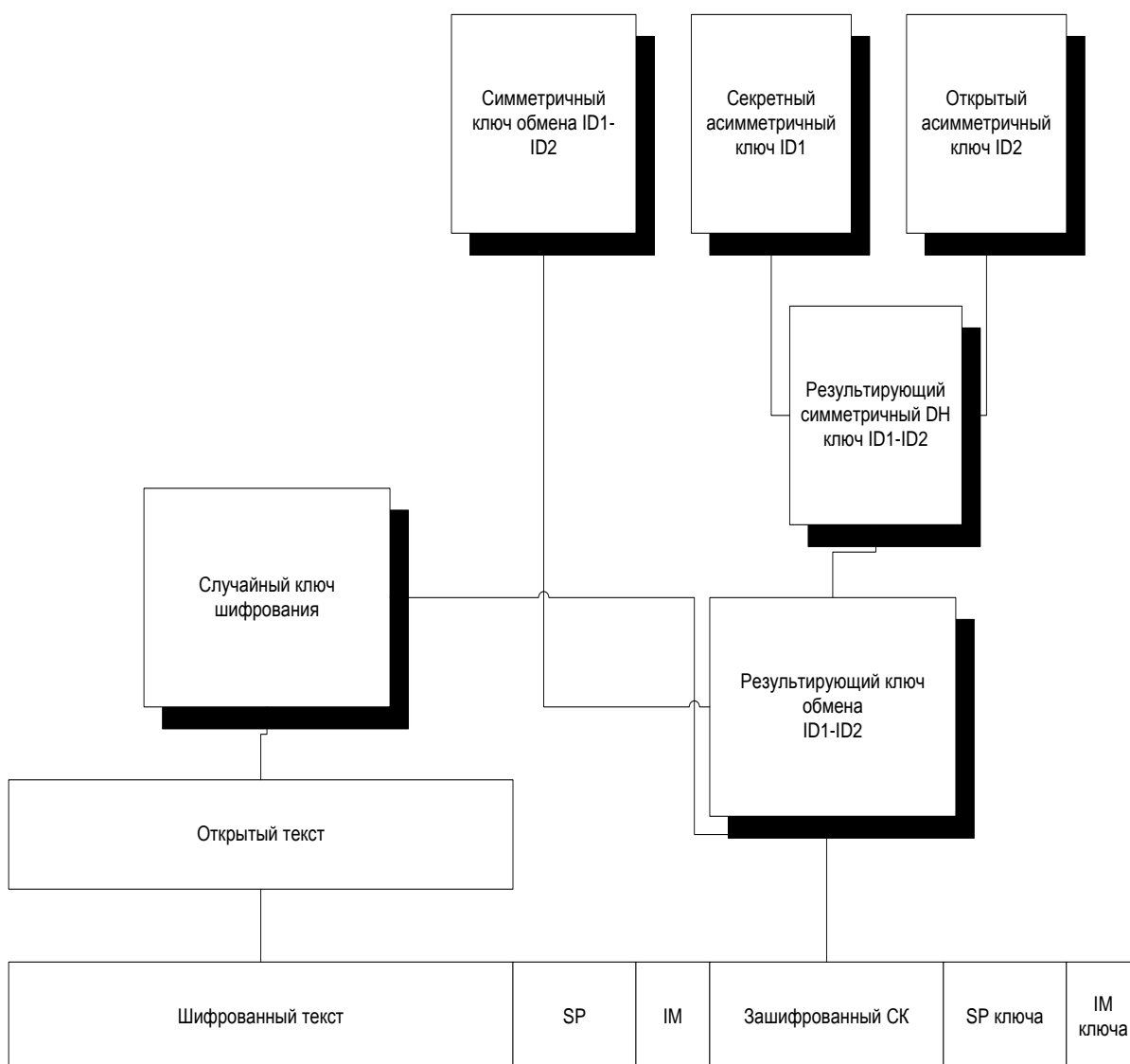
Рис. 9. Шифрование на прикладном уровне
