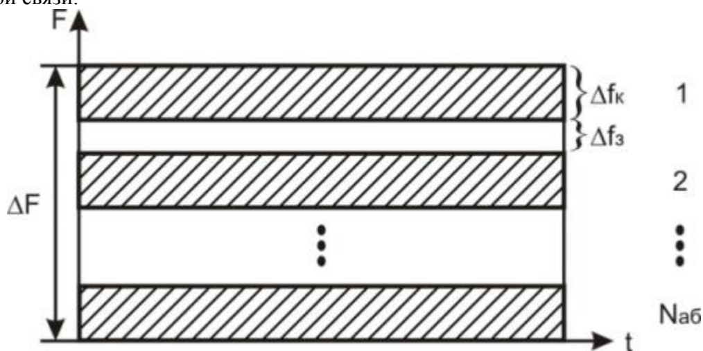
Рис. 1.4.1. Принцип частотного разделения каналов
