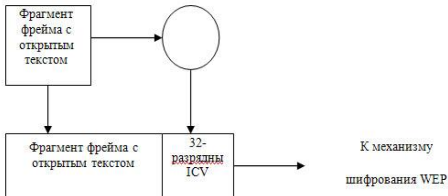
Рис. 1.5.6. Диаграмма функционирования механизма ICV
