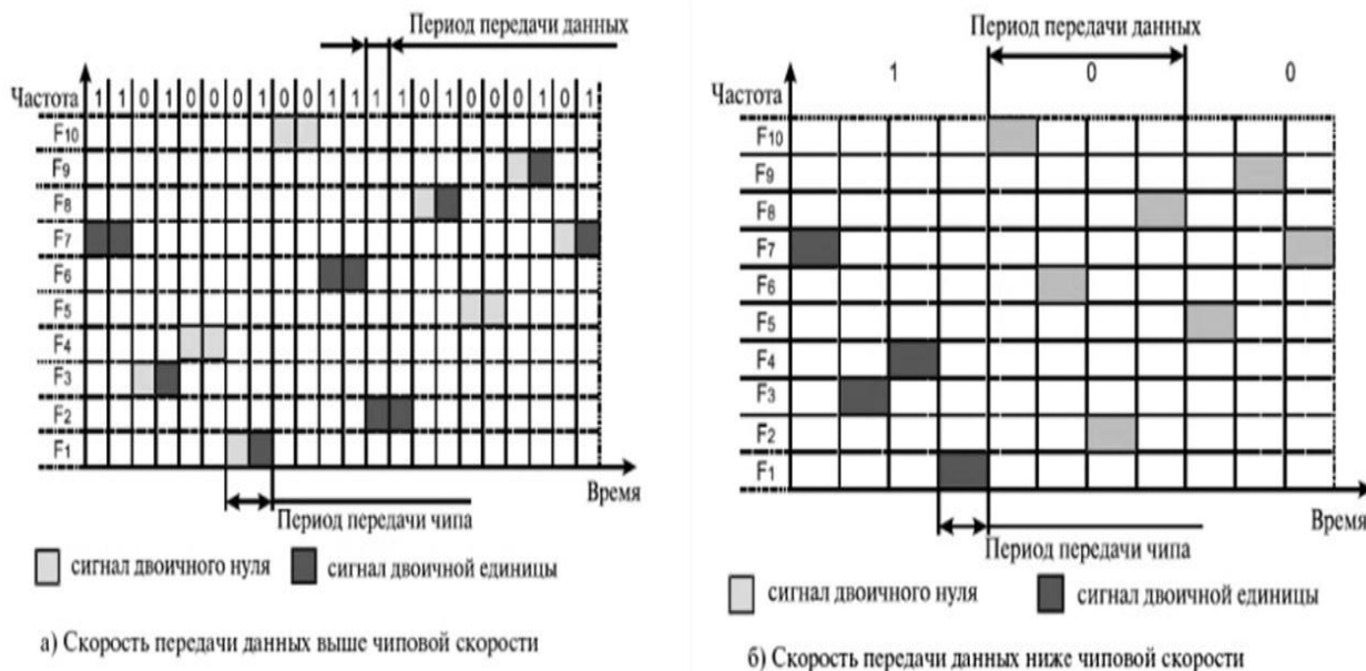
Рис. 1.4.4. Соотношение между скоростью передачи данных и частотой смены подканалов
