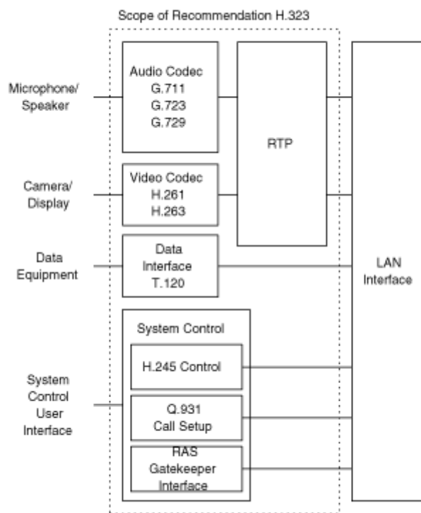
Рис.2. Структура терминала H.323.
