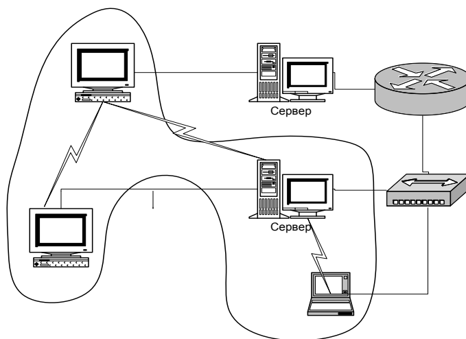
Рис. 3. Взаимодействие клиент-сервер VPN
