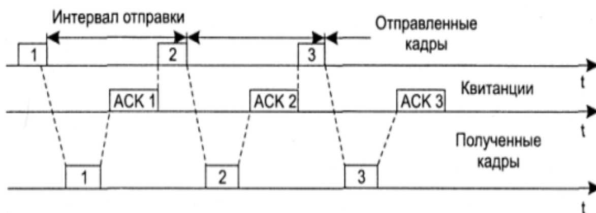
Рис. 1.4.6. Процедура запрос ARQ с остановками
