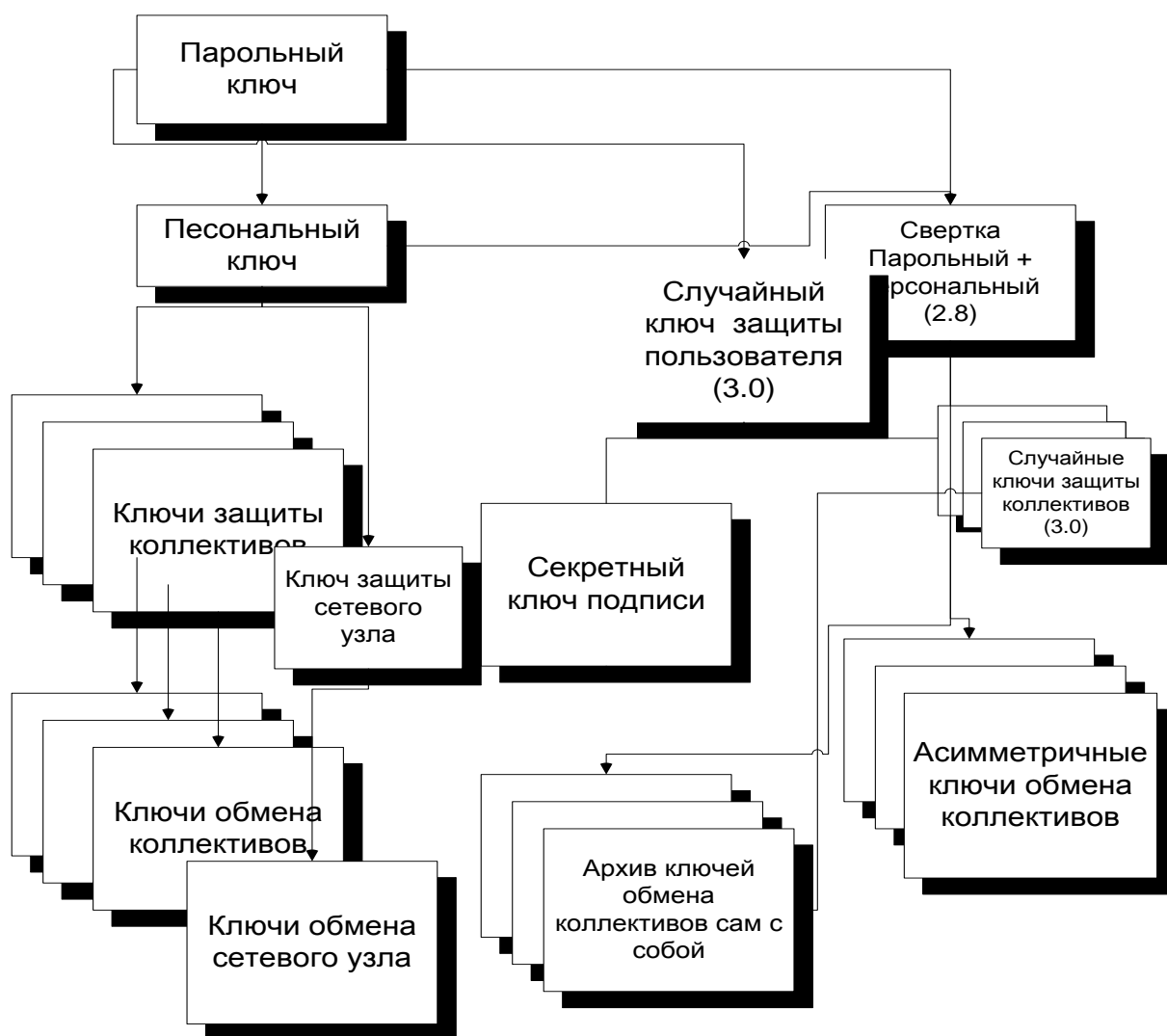
Рис. 7. Виды ключей
