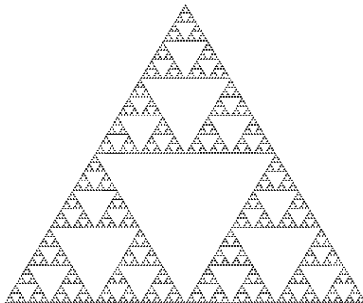
Рис. 3.3.2. Треугольник Серпинского
