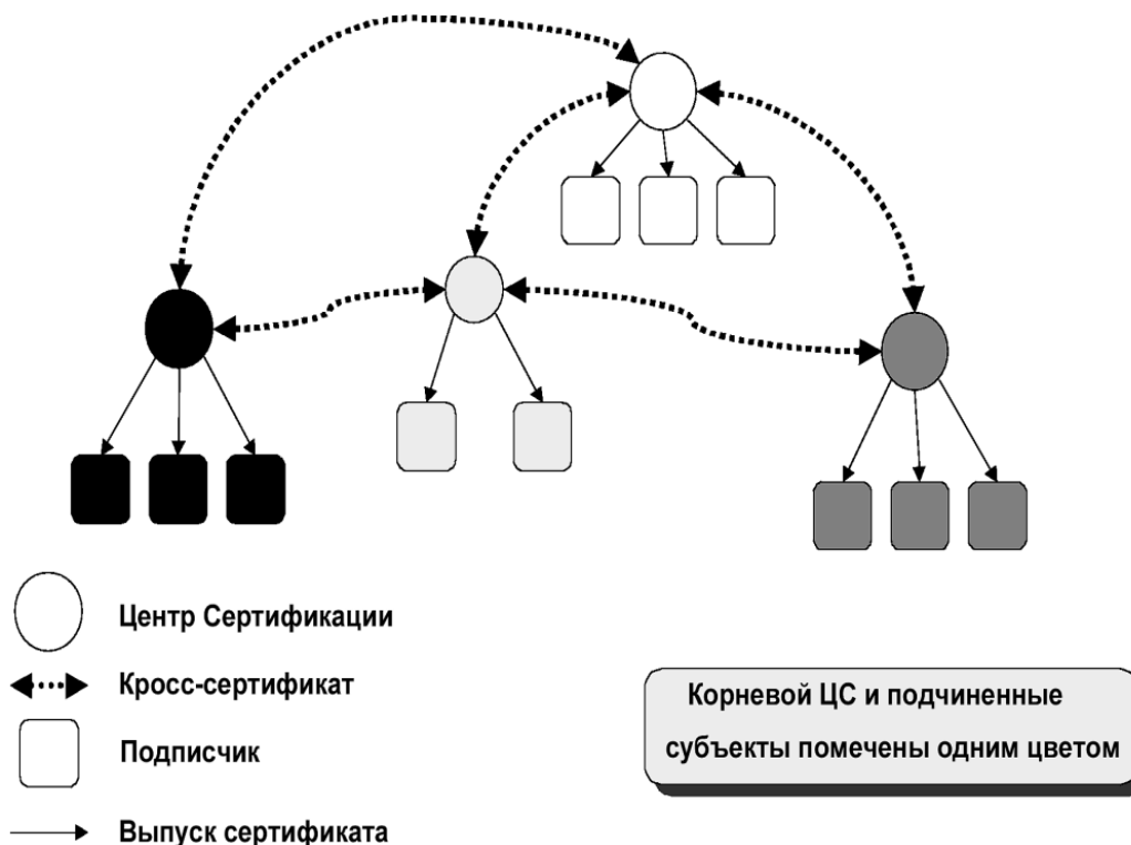
Рис. 13. PKI с топологией узловой сети
