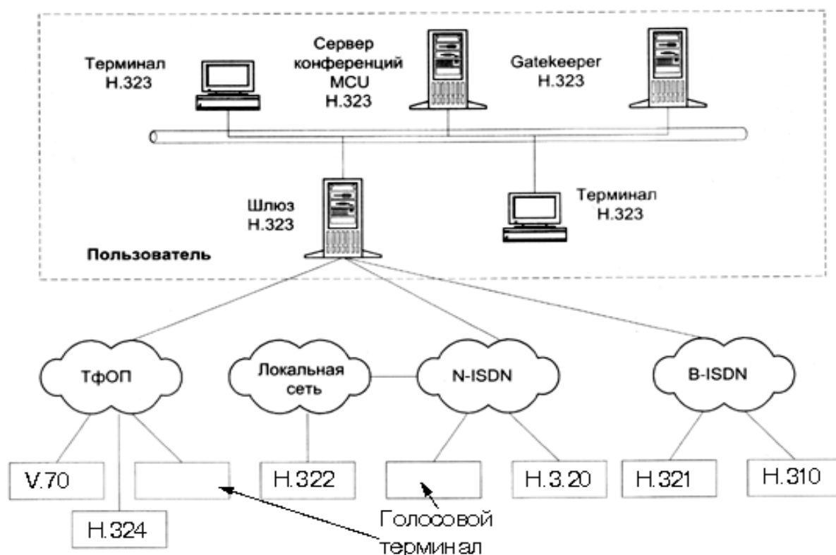
Рис. 2. Конфигурация сети на базе стандарта H.323
