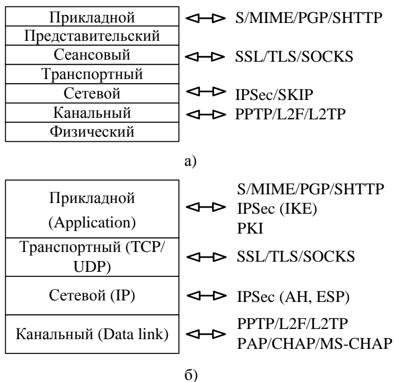
Рис. 2.3. Уровни защищенных каналов
