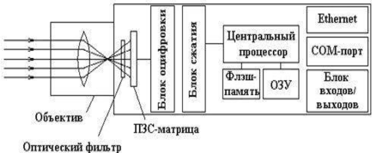
Рис. 2.4.1. Устройство IP-камеры
