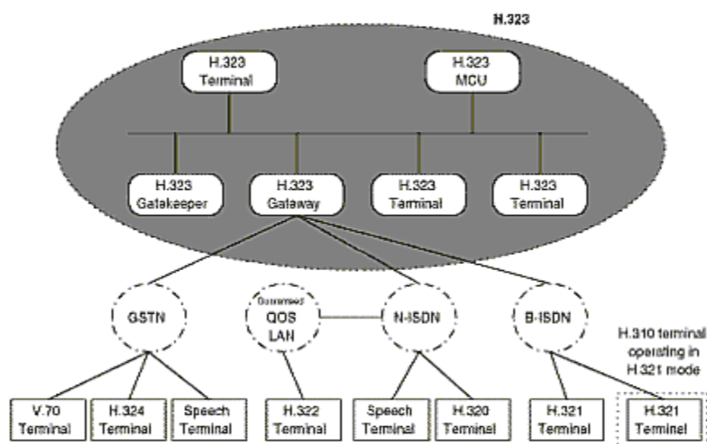
Рис.1. Базовая архитектура стандарта H.323
