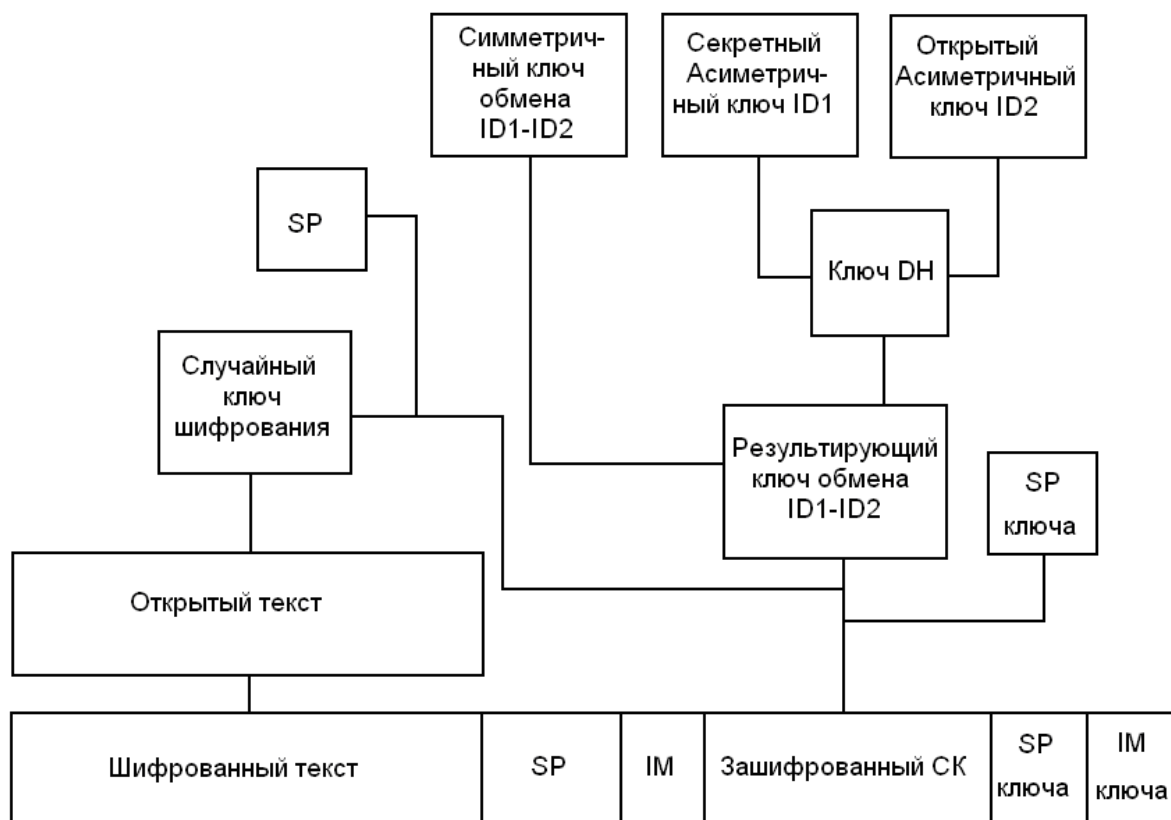
Рис. 22. Алгоритм шифрования на прикладном уровне
