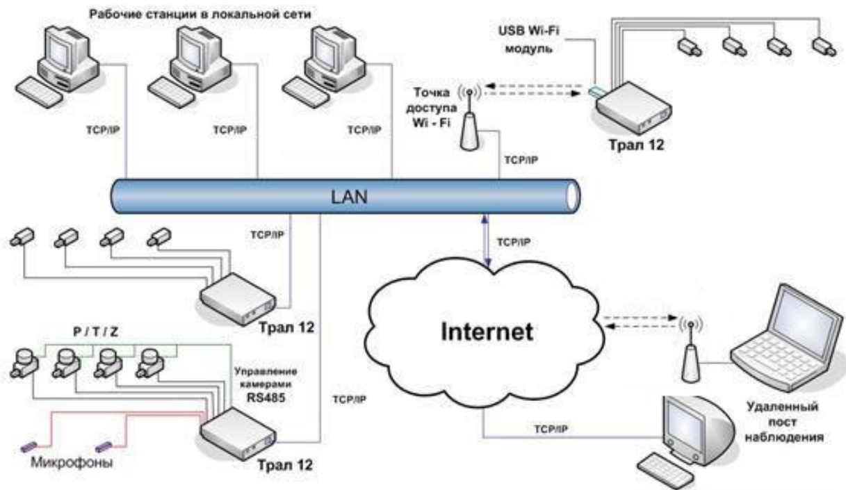
Рис. 2.2.2. Система видеонаблюдения интегрированная в локальную сеть учреждения
