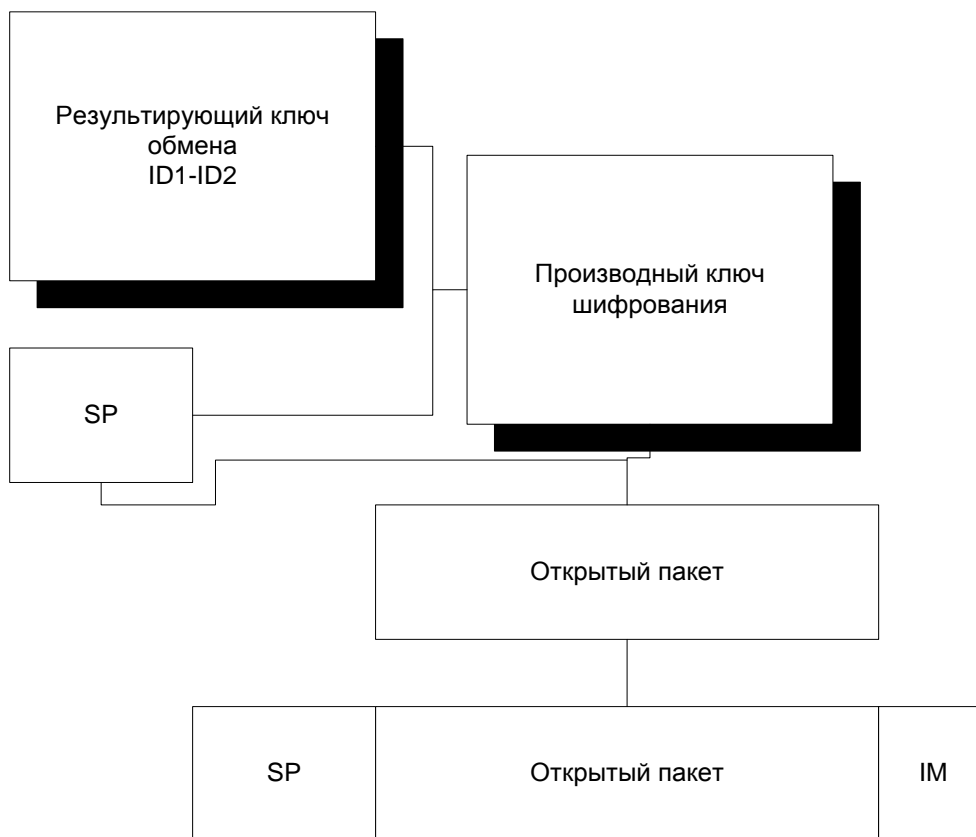
Рис. 10. Шифрование на сетевом уровне
