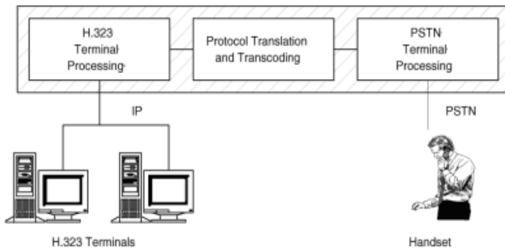
Рис.3. Мультимедиа шлюз H.323/PSTN.
