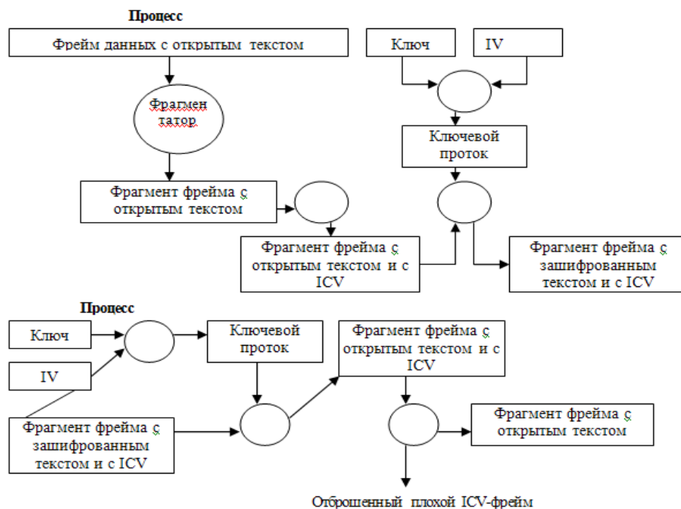
Рис. 1.5.5. Процесс шифрования и дешифрования
