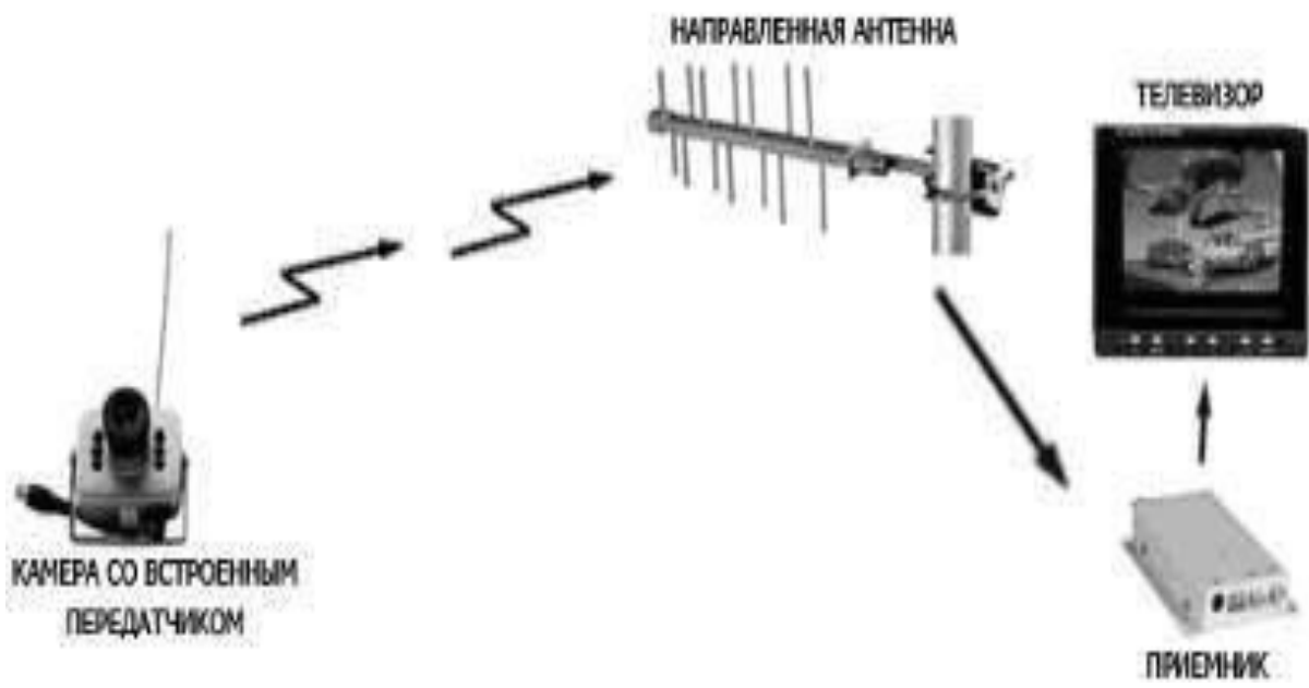
Рис. 2.3.3. Направленная антенна на приемнике
