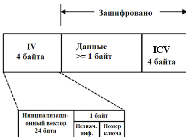
Рис. 1.5.4. Фрейм, зашифрованный по алгоритму WEP.
