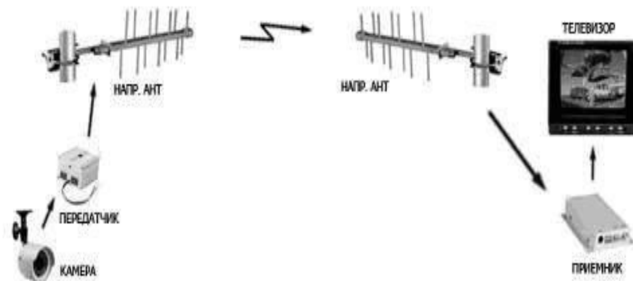
Рис. 2.3.5. Направленная антенна на передатчике и направленная антенна на приемнике
