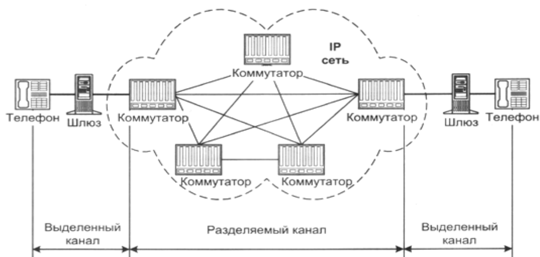
Рис. 1. Соединение в сети с коммутацией пакетов
