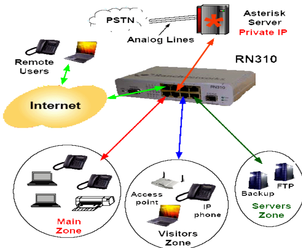
Рис. 21. Пример решения с RN310
