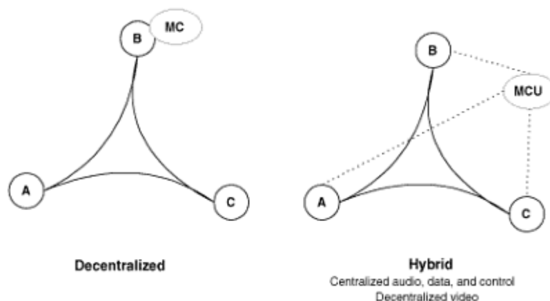
Рис. 6. Схемы децентрализованной и смешанной организаций конференции в H.323.
