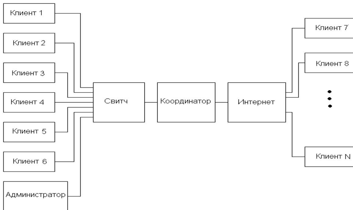
Рис. 83. Защищенная сеть на базе технологии ViPNet Custom
