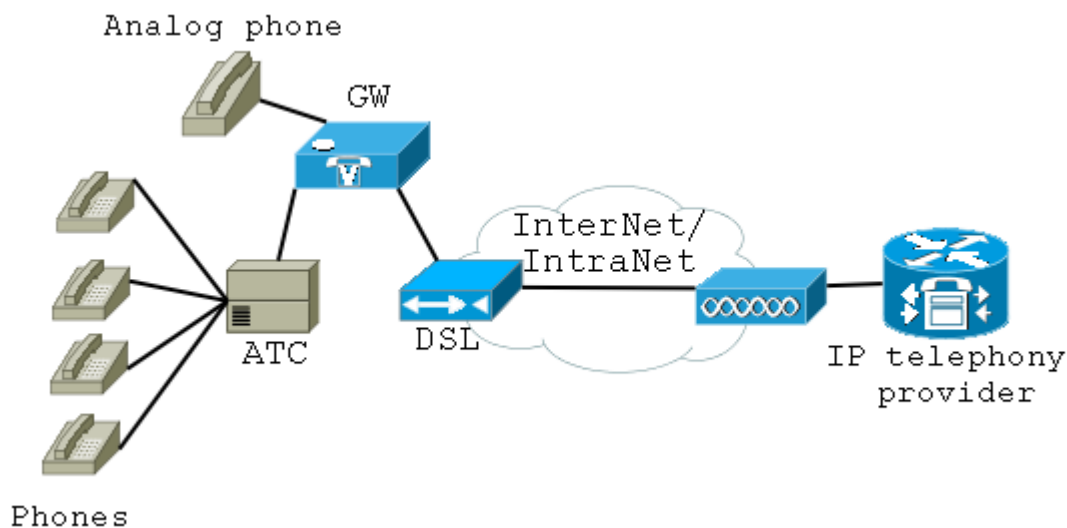
Рис. 6 Схема реализации IP-телефонии при подключении к серверу провайдера
