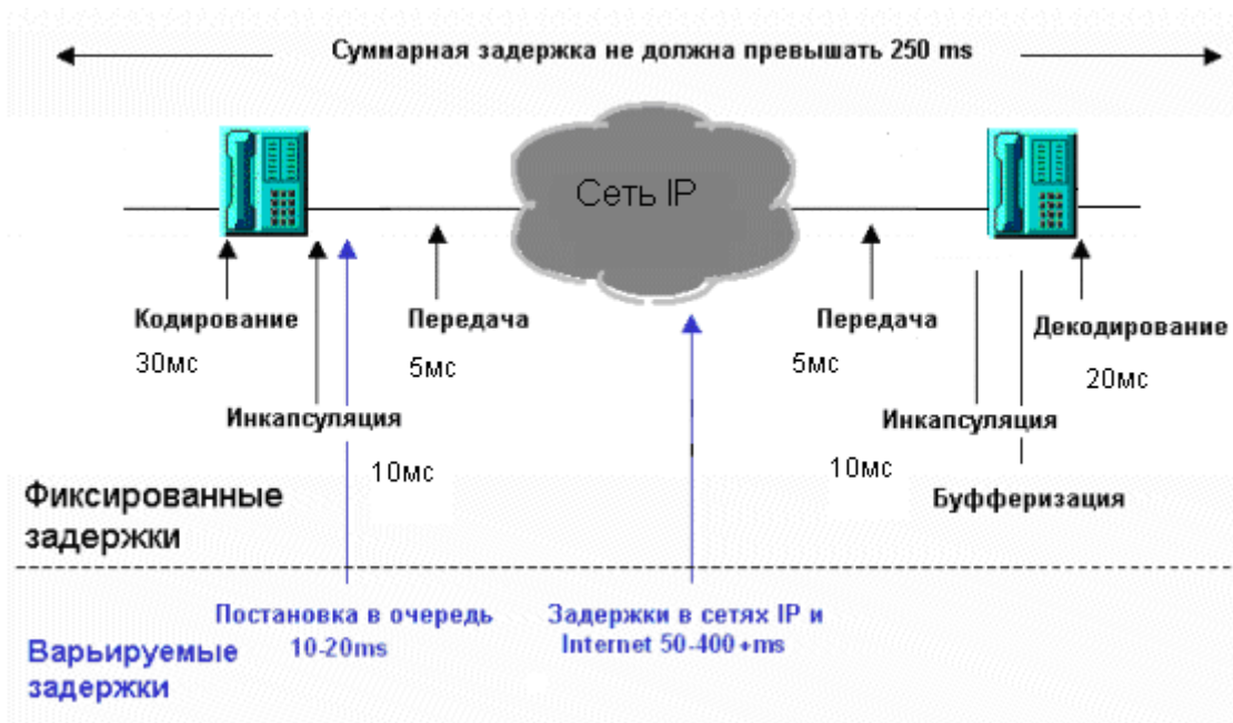
Рис. 14. Составляющие задержки в сети IP-телефонии
