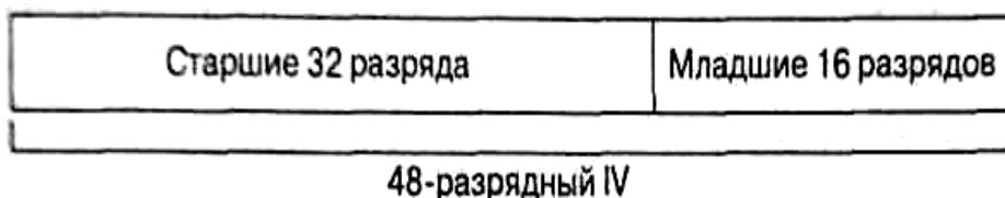
Рис. 1.6.4. Разбиение на части IV для использования при пофреймовом изменении ключа
