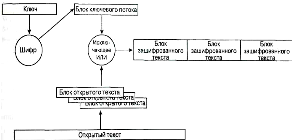
Рис. 1.5.1. Работа поточного шифра
