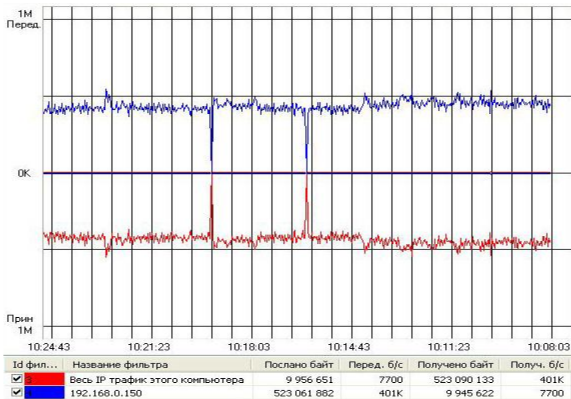
Рис. 3.5.3 Нагрузка на сеть при передаче статичного изображения
