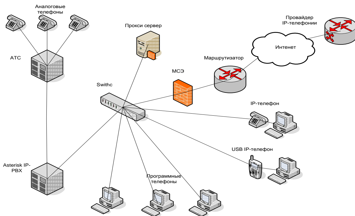
Рис. 13. Структура сети IP-телефонии на основе Asterisk IP PBX
