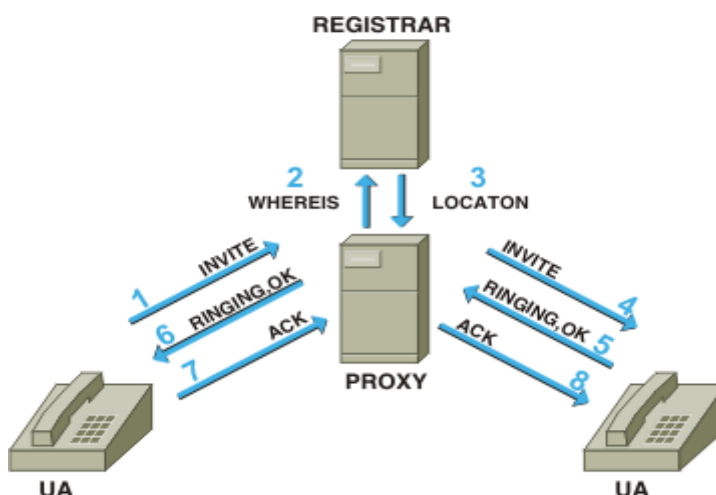
Рис. 4. Схема сигнализации по протоколу SIP
