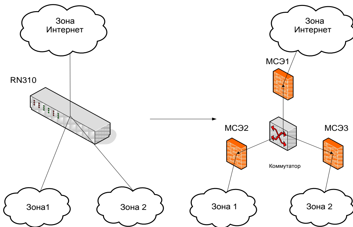
Рис. 24. Логическое изображение продукта RN310 для сетевой топологии с 3-мя зонами безопасности
