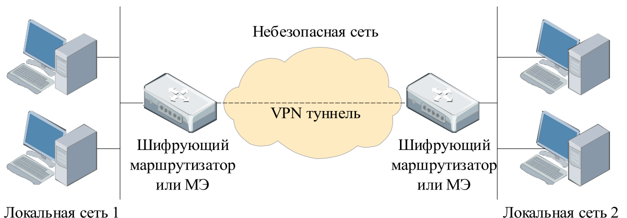
Рис. 2.1. Структура VPN
