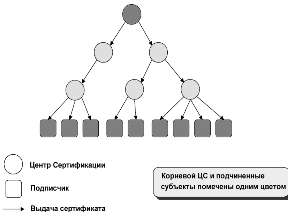
Рис. 11. Иерархическая PKI
