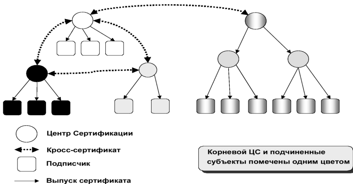
Рис. 14. Гибридная PKI
