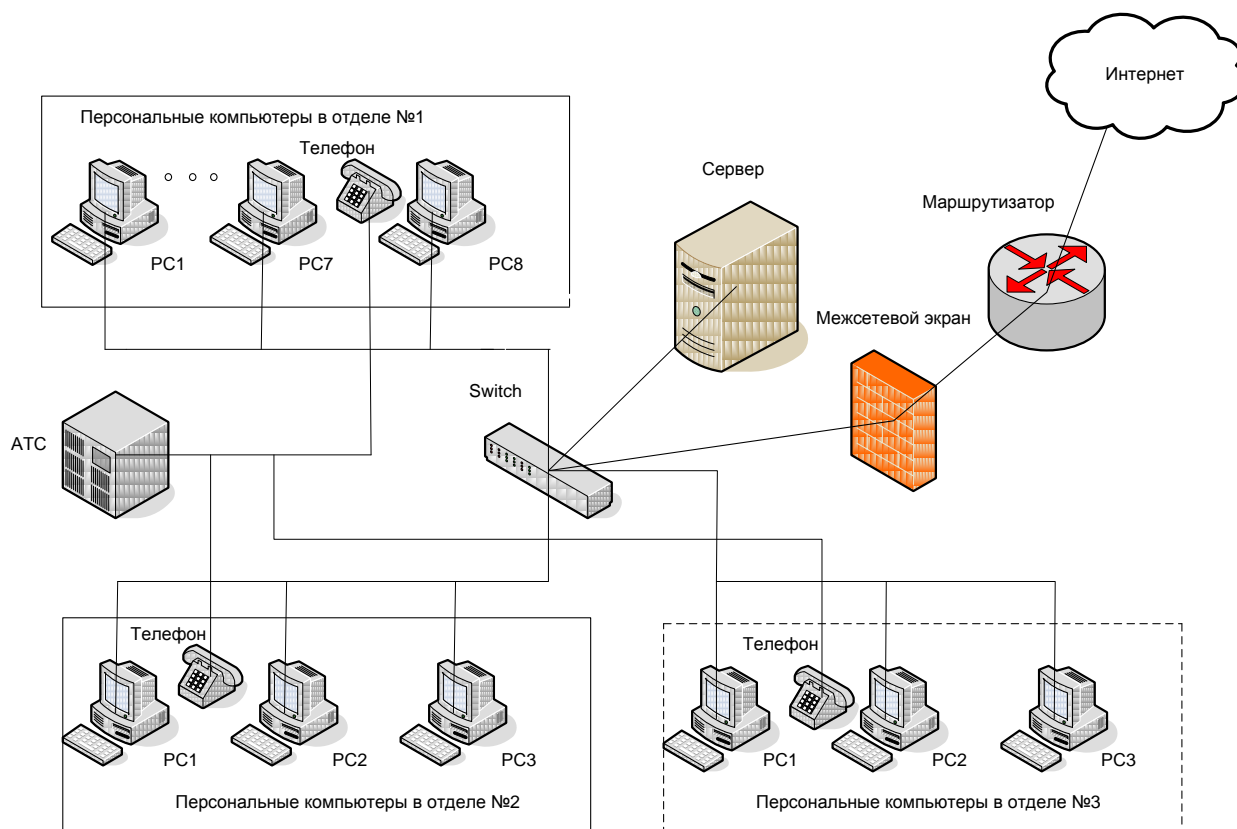
Рис. 7. Структура подсети НПФ «Микран» до внедрения IP-телефонии
