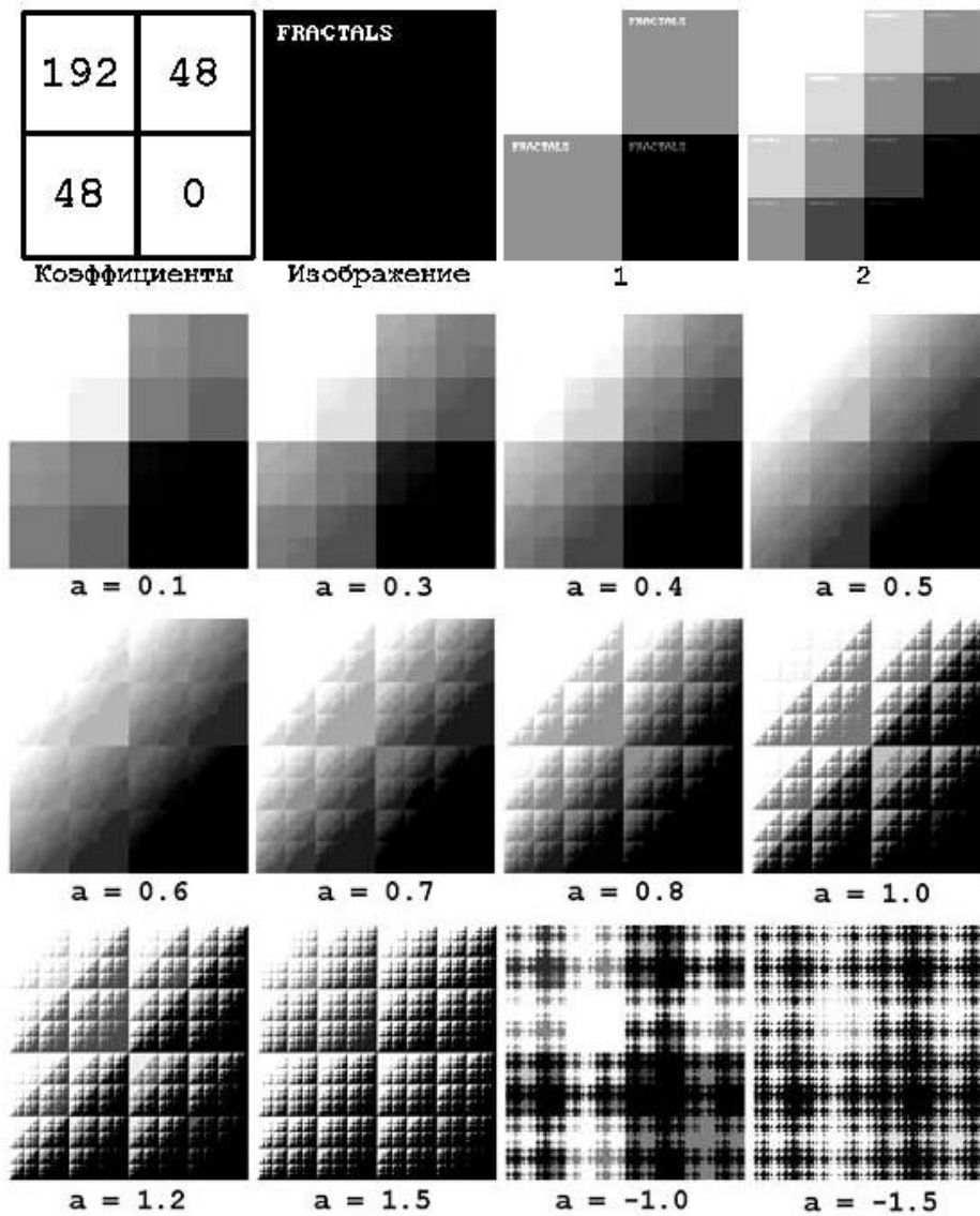
Рис. 3.3.1. Итерации восстановления изображения из кода
