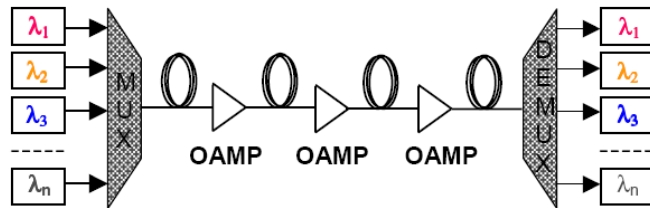
Рис. 1. Структурная схема ВОСП со спектральным уплотнением
