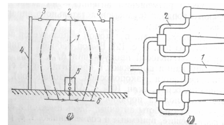
Рис. 1. Антенны: а – линейная проволочная; б – поверхностных волн
