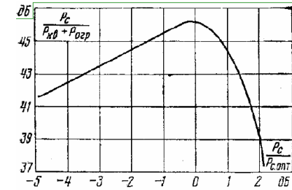
Рис. 1. Зависимость отношения сигнал-шум от уровня сигнала
