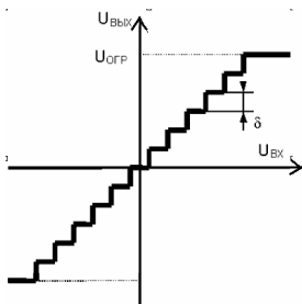
Рис. 5. Амплитудная характеристика равномерного квантователя.
