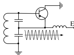
Рис.2. Гармонический LC-генератор
