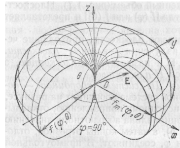
Рис 7. Пространственная (объемная) ДН диполя Герца
