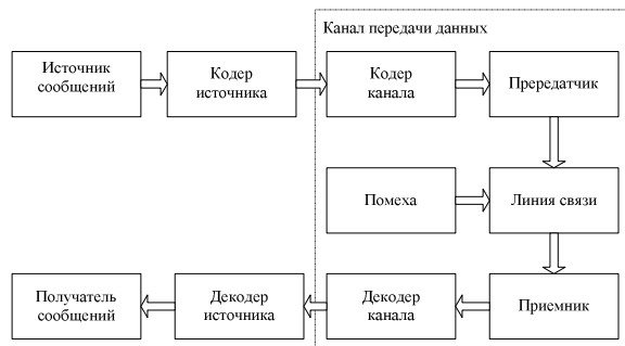
Рис. 1. Обобщенная структурная схема системы передачи дискретных сообщений
