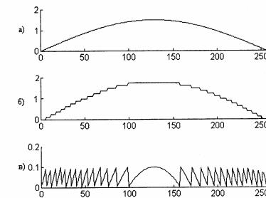
Рис. 1. Сигнал до квантования (а), сигнал после квантования (б), ошибка квантования (в)
