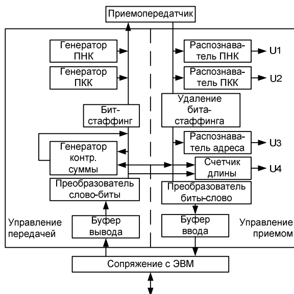
Рис. 12. Управление передачей кадров
