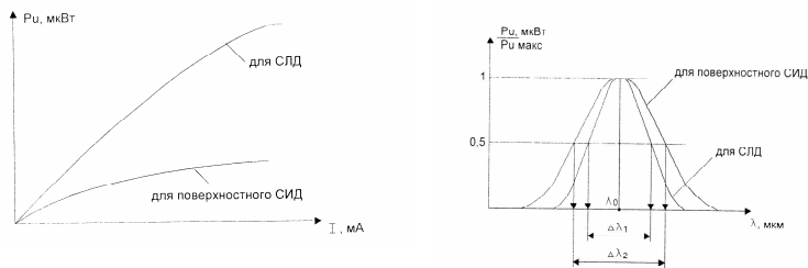
Рис. 1. Ватт-амперная характеристика СИД
