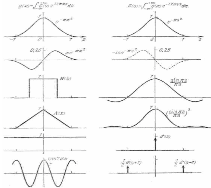
Рис. 1. Спектры некоторых распространенных сигналов.
