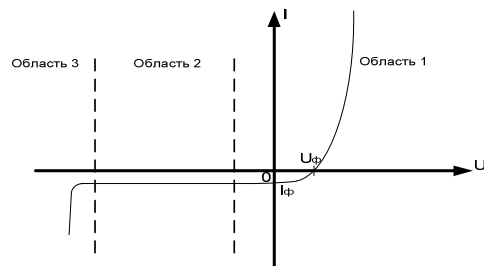
Рис.2 Вольт-амперная характеристика p-n перехода.
