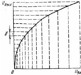
Рис.3. Характеристика компрессии
