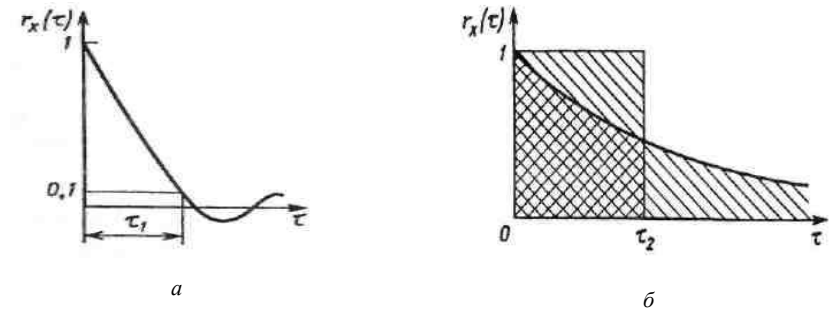
Рис.1. Определение интервала корреляции.
