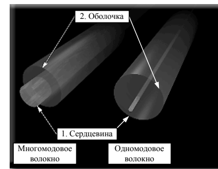
Рис. 1. Структура оптических многомодовых и одномодовых волокон
