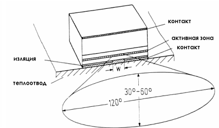
Рис. 2. Конструкция торцевого СИД
