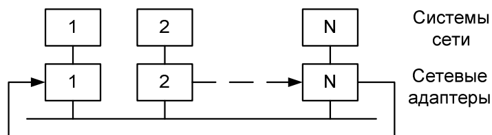
Рис. 5. Эстафетный доступ в ЛВС
