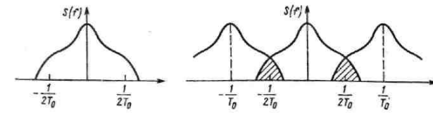
Рис.4. Спектр дискретизированных сигналов
