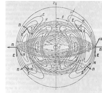
Рис. 2. Поля излучения диполя Герца
