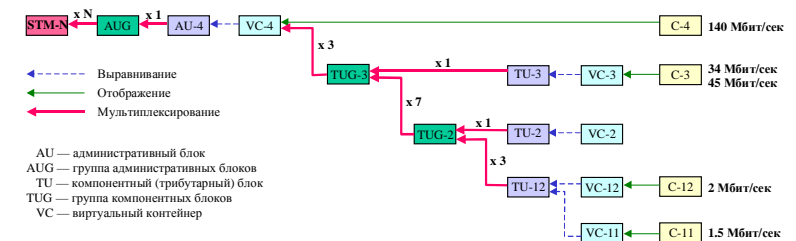
Рис. 4. Схема мультиплексирования PDH сигналов в технологии SDH
