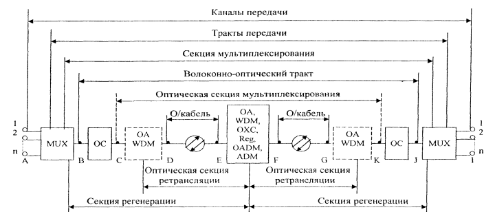
Рис. 1. Структурная схема волоконно-оптической системы передачи
