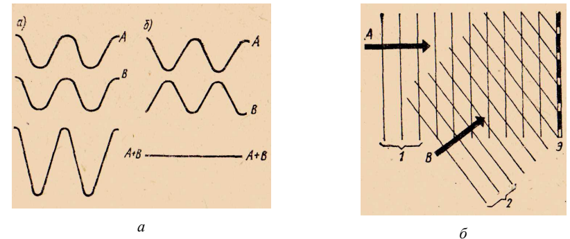
Рис. 3. Интерференция двух плоских волн на экране:
