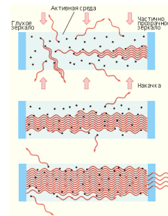
Рис.2. Развитие лавинообразного процесса генерации в лазере.
