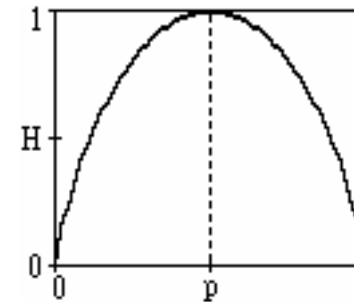
Рис.1. Зависимость энтропии от вероятности сообщения
