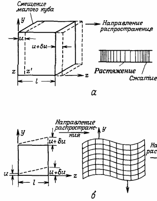
Рис. 1. а - распространение продольной волны; б - распространение поперечной (сдвиговой) волны.
