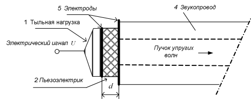
Рис. 1. Структура резонансного преобразователя для объемных акустических волн.
