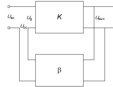
Рис.1. Усилитель с обратной связью по напряжению.
