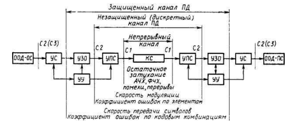
Рис. 1.1. Структурная схема системы аппаратуры передачи данных (СПД)
