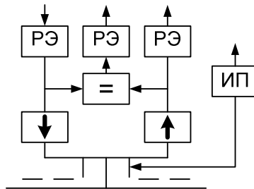
Рис. 10. Развязывающие элементы на оптронах
