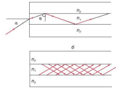
Рис. 3. Распространение света в плоском волноводе.
