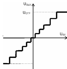
Рис. 6. Амплитудная характеристика неравномерного квантователя.
