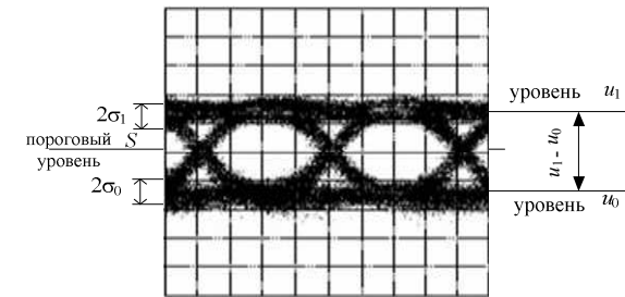
Рис.1. Глаз-диаграмма оптического сигнала
