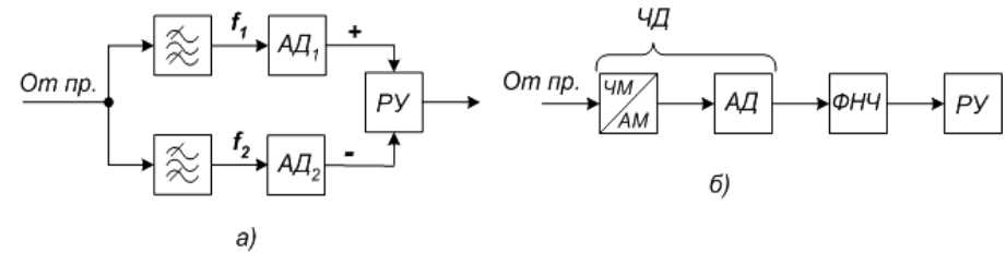
Рис. 1. Структурные схемы детекторов ЧМ сигналов
