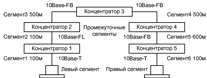
Рис. 15. Пример сети для расчета PDV
