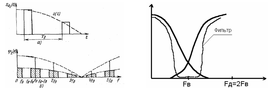
Рис. 4. Амплитудно-импульсная модуляция второго рода: а) отсчеты аналогового сигнала; б) спектр последовательности отсчетов в) АЧХ фильтра
