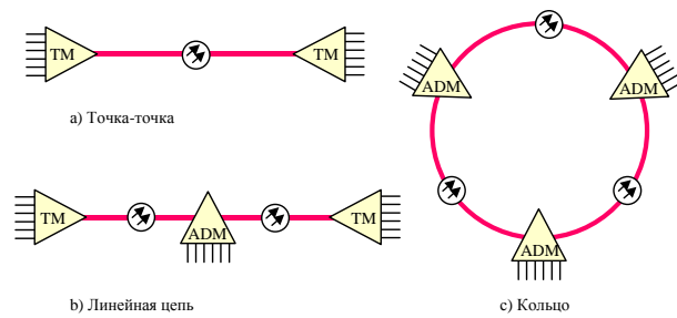
Рис. 1. Базовые топологии SDN сетей
