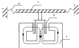
Рис. 1. Электродинамический преобразователь
