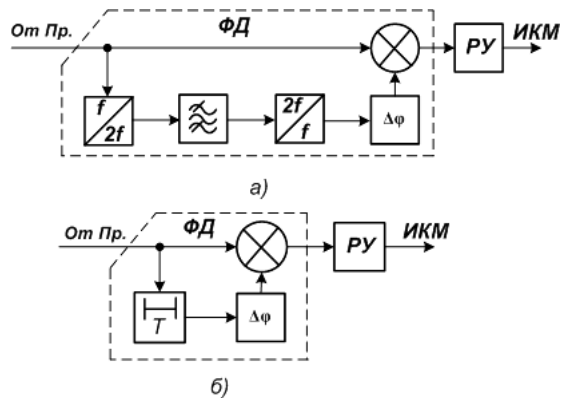
Рис. 1. Структурные схемы детекторов ФМ сигналов
