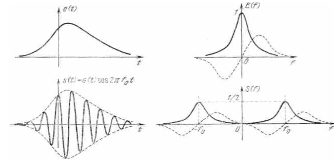
Рис. 2. Спектр синусоидального сигнала, модулированного по амплитуде.
