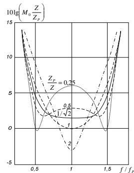
Рис. 2. Система преобразователь - звукопровод.
