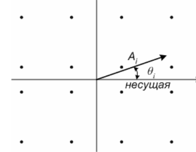
Рис. 2. Расположение сигнальных точек 16-кратной АФМ в фазово-амплитудном пространстве
