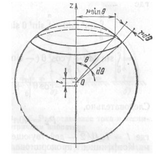
Рис. 3. К расчету сопротивления излучения диполя Герца
