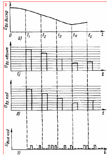
Рис. 2. Временные диаграммы работы импульсно-кодового модулятора: а) входной аналоговый сигнал; б) последовательность отсчетов; в) последовательность квантованных отсчетов; г) последовательность кодовых групп
