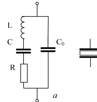
Рис. 1. Кварцевый резонатор: а) эквивалентная схема; б) обозначение
