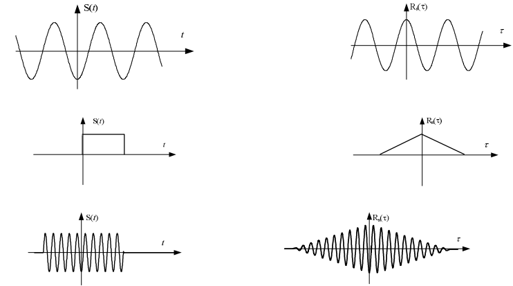
Рис. 1. Автокорреляционные функции некоторых типов детерминированных сигналов.
