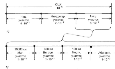
Распределение коэффициента ошибок в ОЦК:
