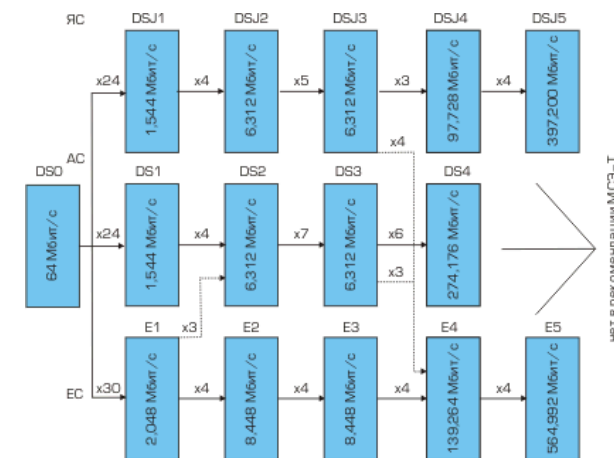
Рис.3. Плезизохронная цифровая иерархия PDH
