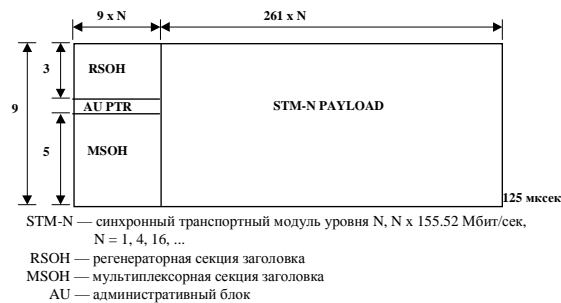
Рис.3 Структура фрейма STM-N
