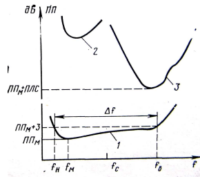
Рис. 3. Типичная форма частотных зависимостей потерь преобразования основного (1) и неосновных (2 и 3) типов излучаемых акустических волн
