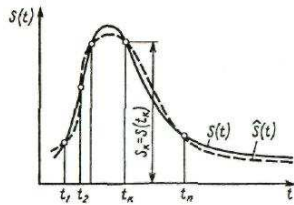
Рис.1. Представление сигнала отсчетами
