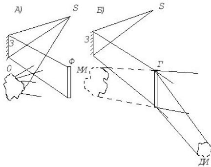
Рис. 1. – Схемы получения голограммы(А) и восстановления волнового фронта(Б) S - источник света; O - объект, φ - фотопластинка; Γ - голограмма; З — зеркало; МИ - мнимое изображение; ДИ - действительное изображение
