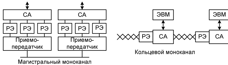
Рис. 9. Развязывающие элементы в ЛВС
