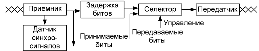
Рис. 11. Приемопередатчик кольцевой ЛВС
