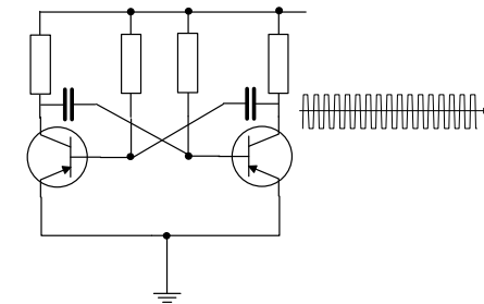
Рис.1. Схема мультивибратора
