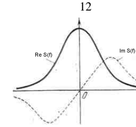
Рис. 1.16. Спектр действительного сигнала.
