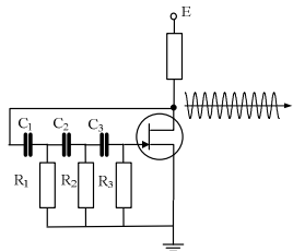
Рис.1. Гармонический RC-генератор
