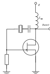
Рис. 1. Схема генератора полевом транзисторе с кварцевой стабилизацией
