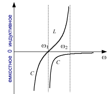
Рис. 2. Частотная характеристика сопротивления кварцевого резонатора
