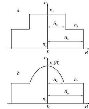
Рис. 4. Распределение показателя преломления по сечению волокна.
