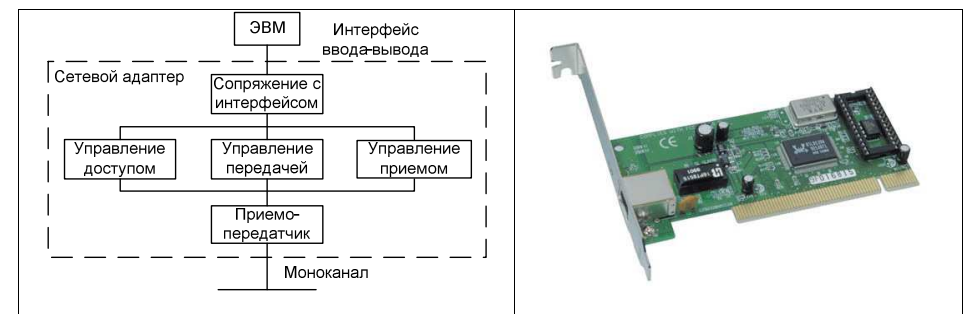
Рис.8. Структура адаптера ЛВС
