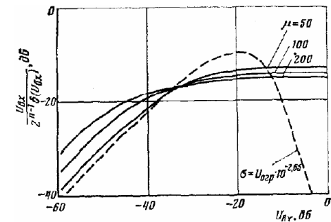
Рис. 4. Зависимость \frac{U_{вх}}{\delta(U_{вх})} от величины входного сигнала.
