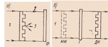
Рис. 8. Схемы получения (а) и восстановления (б) голограммы Габора: / - освещающий пучок; 2 - опорная волна; Я - объектная волна; Ф - фотопластинка; МИ - мнимое восстановленное изображение объекта; Г - голограмма; ДИ - действительное комплексно-сопряженное изображение объекта
