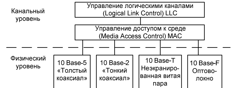
Рис. 14. Соответствие уровней протоколов IEEE и ISO/OSI
