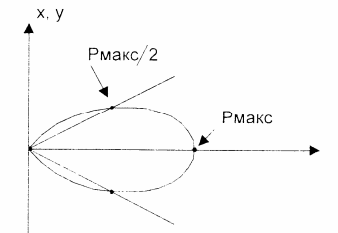
Рис. 3. Угловая расходимость излучения СИД.
