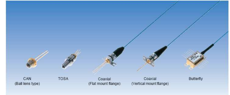
Рис.4. Конструкции лазерных диодов для систем оптической связи
