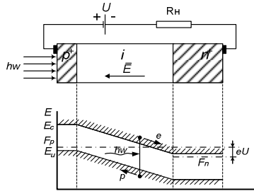
Рис.1 – структура и зонная диаграмма p-i-n-фотодиода
