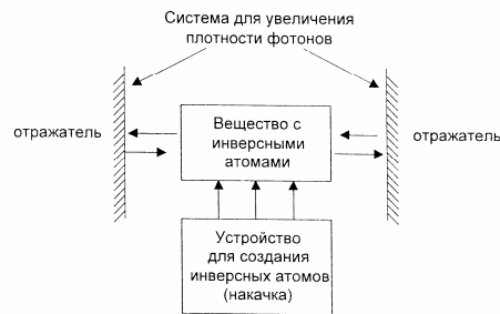
Рис. 3. Обобщенная конструкция лазера
