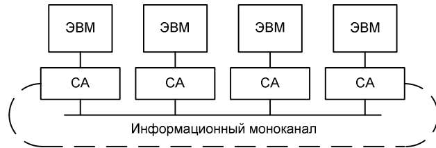
Рис. 3. Сетевые адаптеры и информационный моноканал ЛВС
