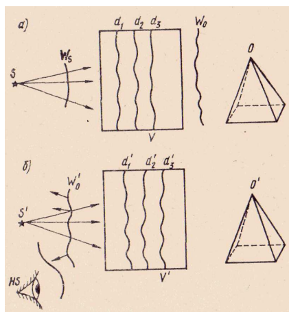
10. Схемы получения (а) и восстановления (б) трехмерной голограммы: S - источник излучения со сплошным спектром; V' - трехмерная голограмма; W 0 ' - волна излучения, восстановленного трехмерной голограммой; O' — восстановленное голограммой объемное изображение объекта, с помощью которого была получена голограмма во время записи.
