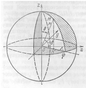
Рис. 6. Сферические координаты точки наблюдения
