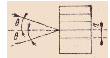
Рис. 9. Интерференционная картина, зарегистрированная в объеме светочувствительной эмульсии.
