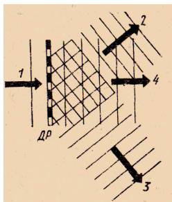
Рис. 5. Получение плоских волн методом дифракции:
