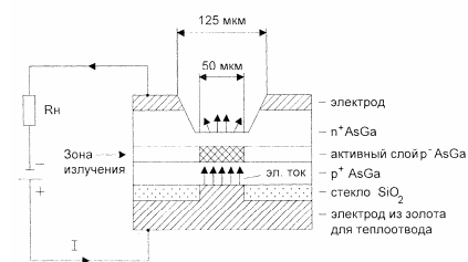
Рис. 1. Конструкция светодиода поверхностного типа (диода Баррасса).
